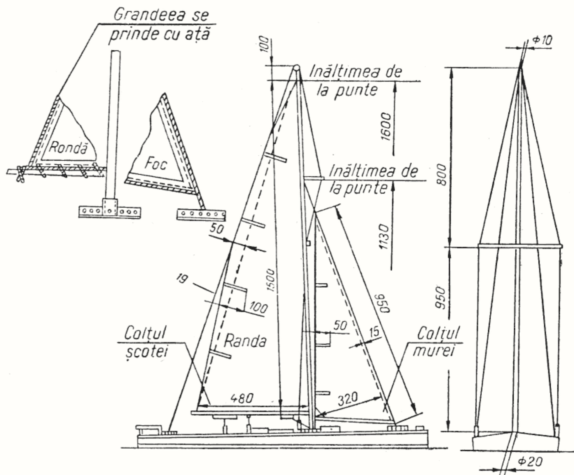
Fig. 90 — Planul velaturii și arborada.
