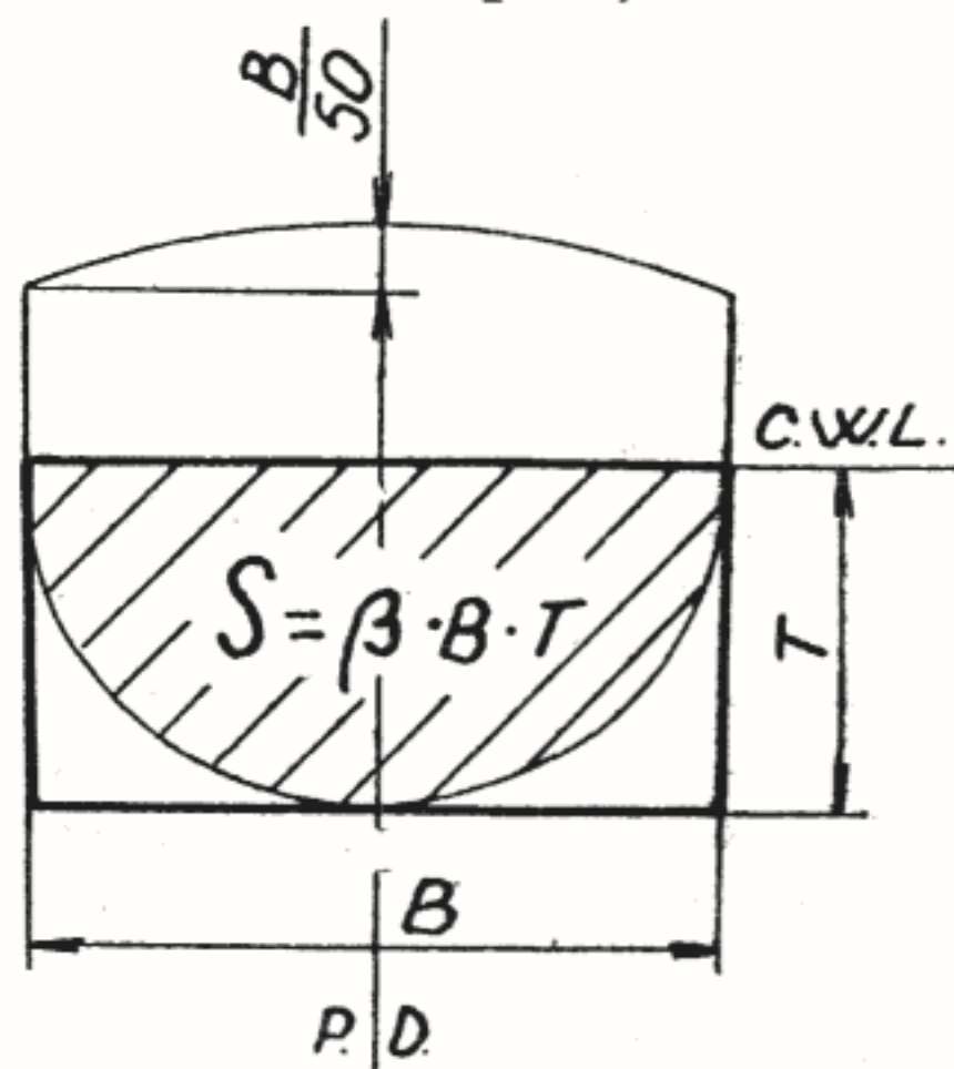
Fig. 16 — Trasajul secțiunii maestre și săgeata punții.
