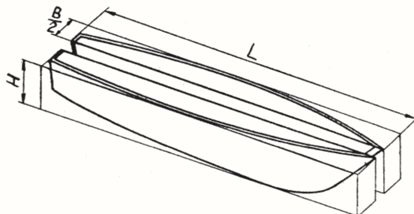
Fig. 46 — Semibărți trasate pentru cioplire.
