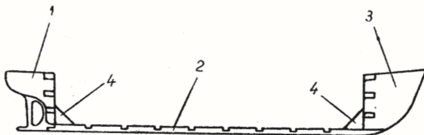
Fig. 28 — 1. Etamboul; 2. chila; 3. etrava; 4. guseu.
