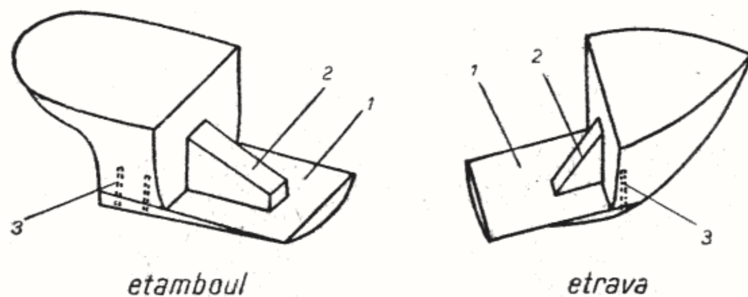
Fig. 30 — Fixarea etravei și etamboului pe chilă (1. chila; 2. guseu; 3. buloane).
