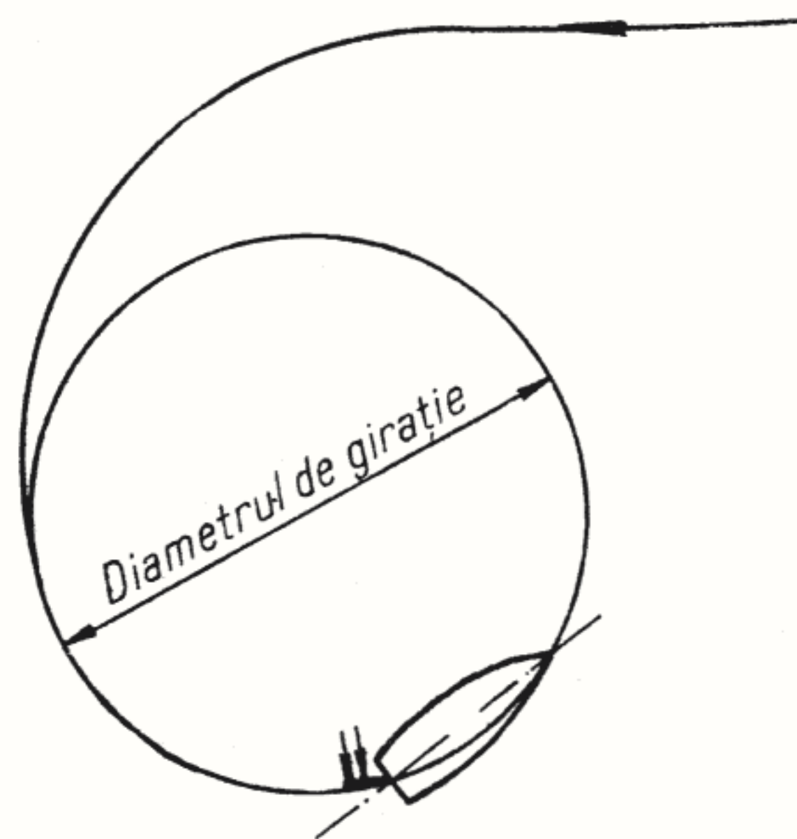
Fig. 8 — Diametrul de girație.
