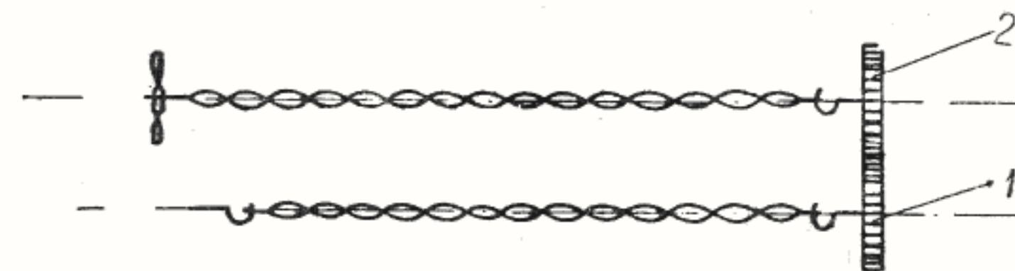
Fig. 50 — Motor cu două fișii de cauciuc și două roți dințate în prova: 1. roata conducătoare; 2. roata condusă.
