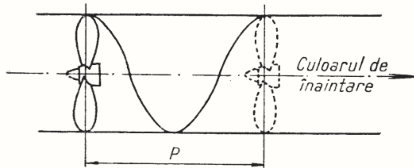
Fig. 59 — Pasul elicei.
