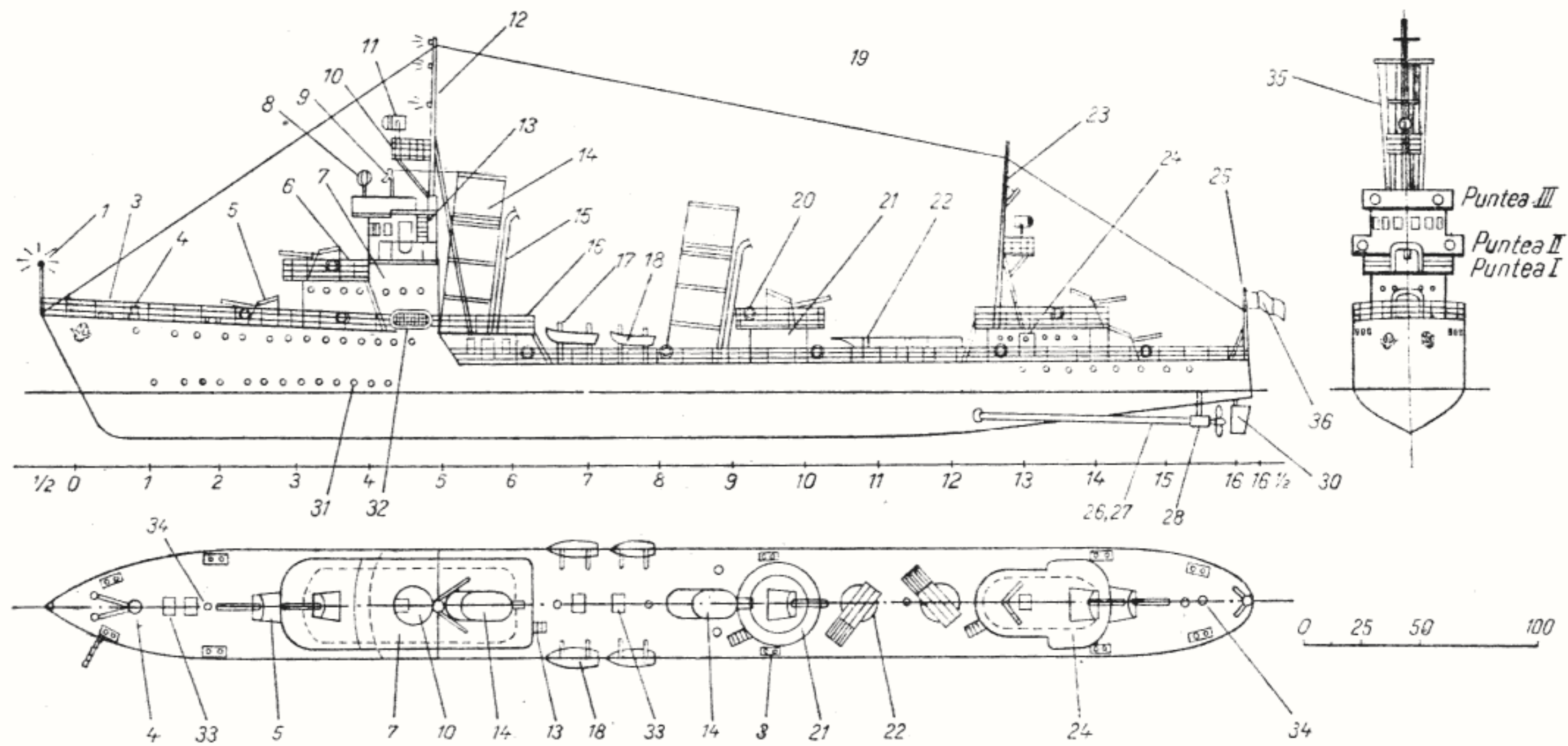
Fig. 67 — Planul de construcție al modelului distrugătorului „Ferdinand”.
