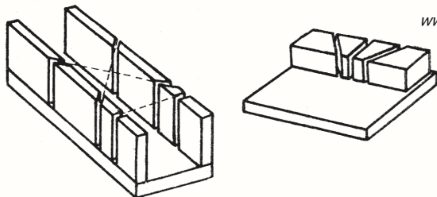
Fig. 2 — Tocuri pentru tăiat lemnul sub unghiuri diferite.
