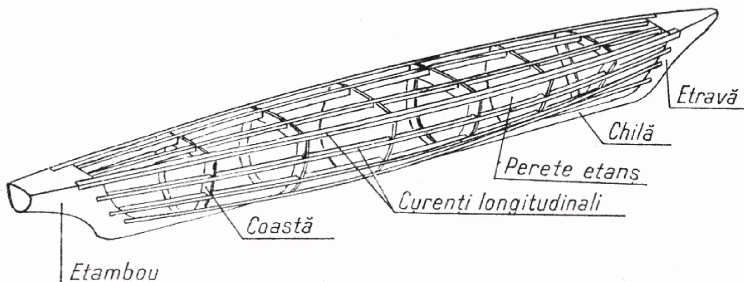
Fig. 32 — Scheletul modelului.
