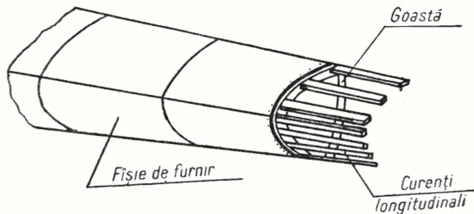
Fig. 34 — Aplicarea învelișului exterior pe scheletul modelului.
