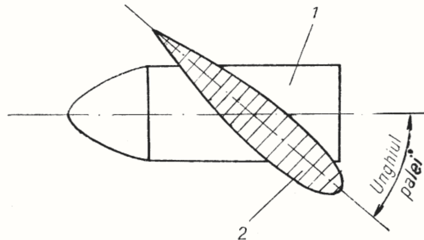
Fig. 60 — Unghiul palei: 1. butucul; 2. pala elicei.
