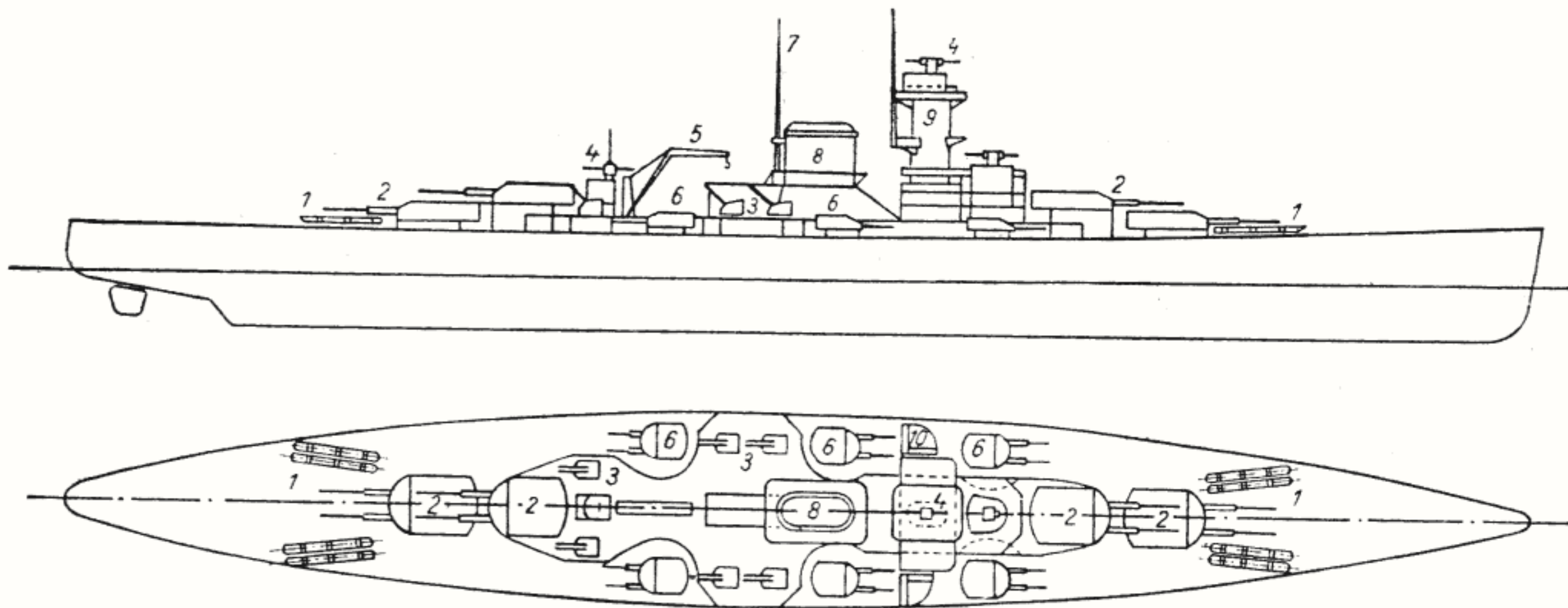
Fig. 5 — Navă de luptă: 1. tuburi lans-torpilor; 2. Armament de artilerie grea; 3. armament de artilerie ușoară (antiaeriană); 4. telemetru; 5. macara simplă; 6. armament de artilerie grea; 7. antenă; 8. coș de fum; 9. turnul de comandă; 10. lumini de poziție.
