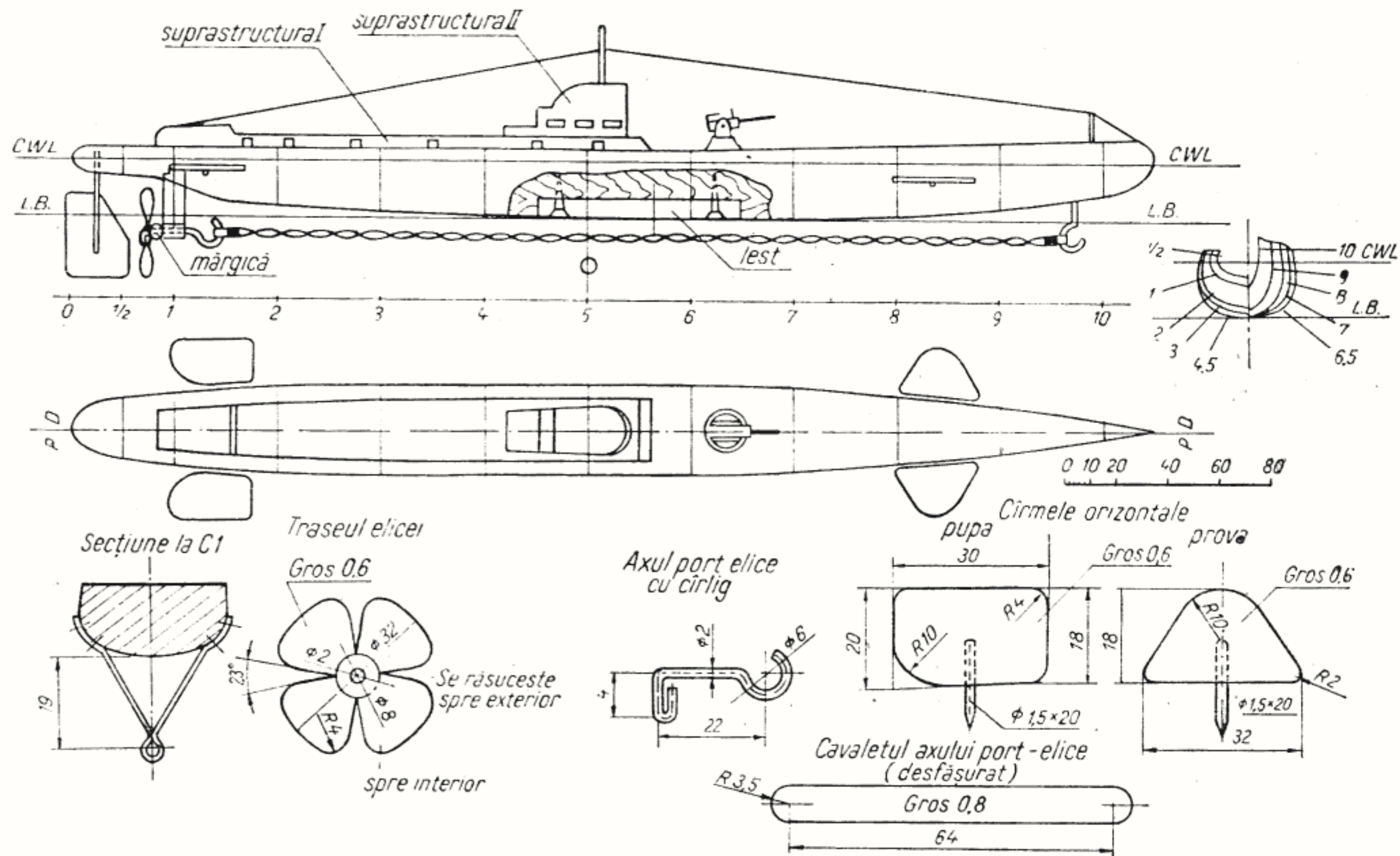
Fig. 65 — Modelul submarinului „Delfinul“.
