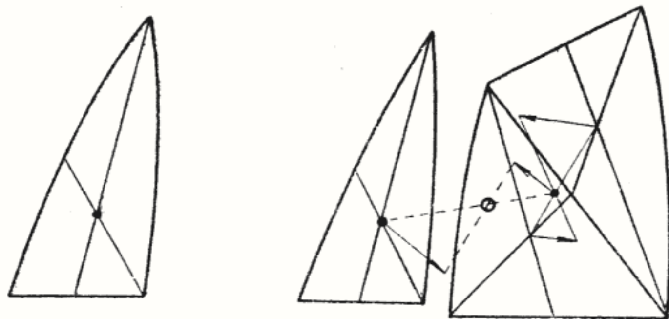
Fig. 23 — Determinarea centrului de velatură.
