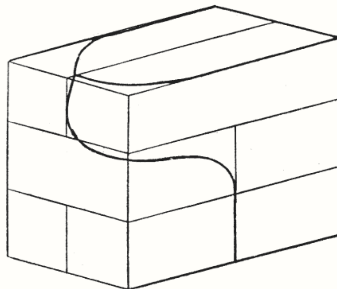
Fig. 26 — Pregătirea lemnului pentru confecționarea etamboului.
