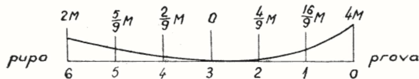
Fig. 14 — Trasajul selaturii punții.
