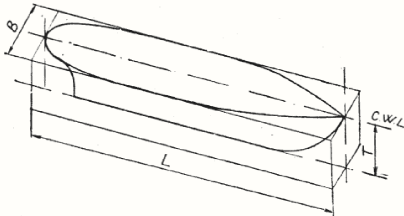
Fig. 10 — Determinarea coeficientului de finețe al corpului.
