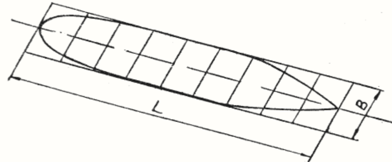
Fig. 11 — Determinarea coeficientului de finețe al liniei de plutire.
