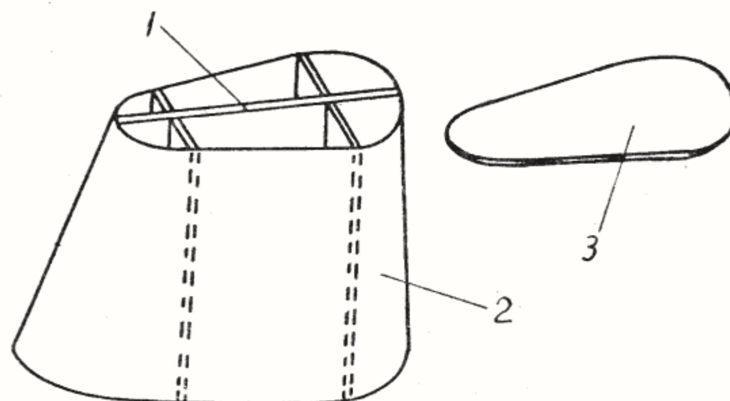
Fig. 43 — Coșul de fum: 1. schelet; 2. înveliș; 3. capac.
