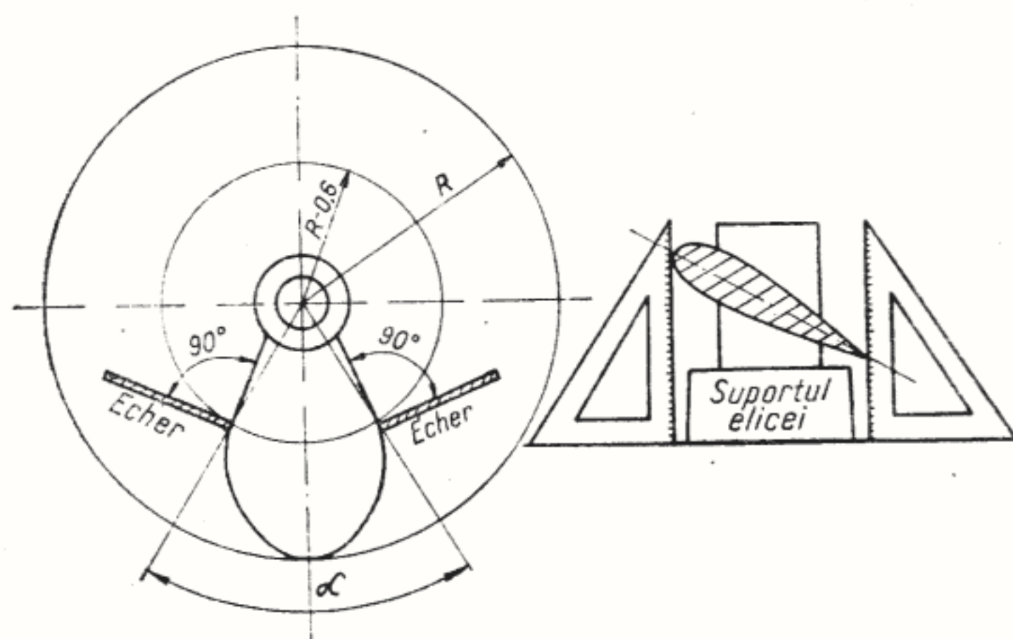
Fig. 61 — Determinarea pasului elicei.
