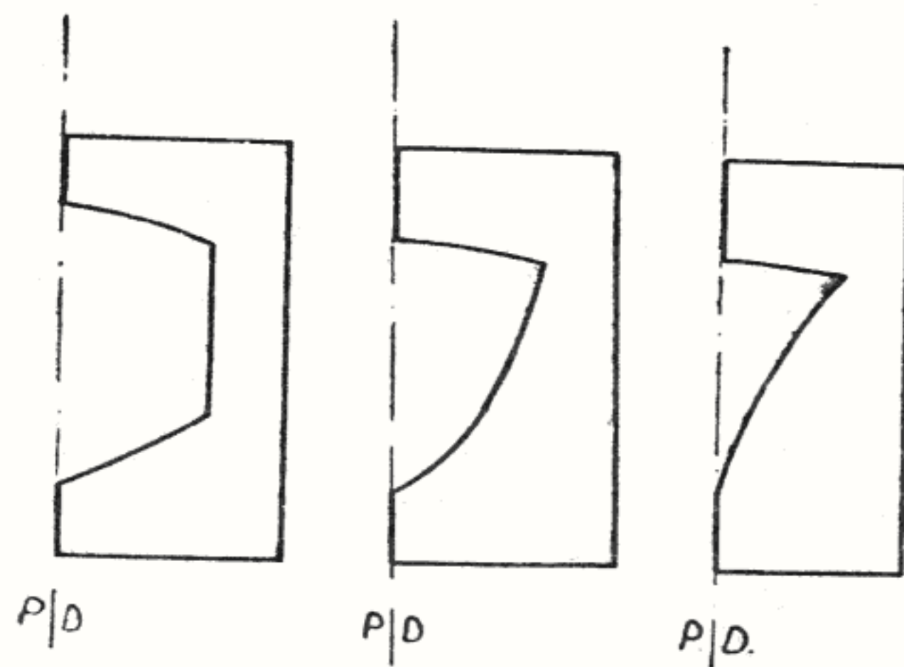
Fig. 33 — Șabloane pentru verificat coastele modelului.
