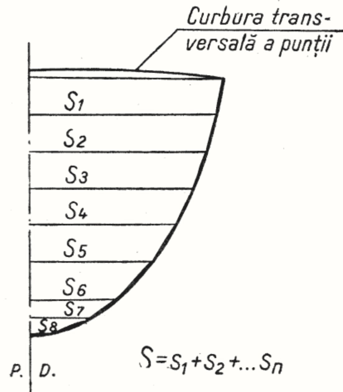
Fig. 12 — Metoda trapezelor pentru calculul suprafețelor.
