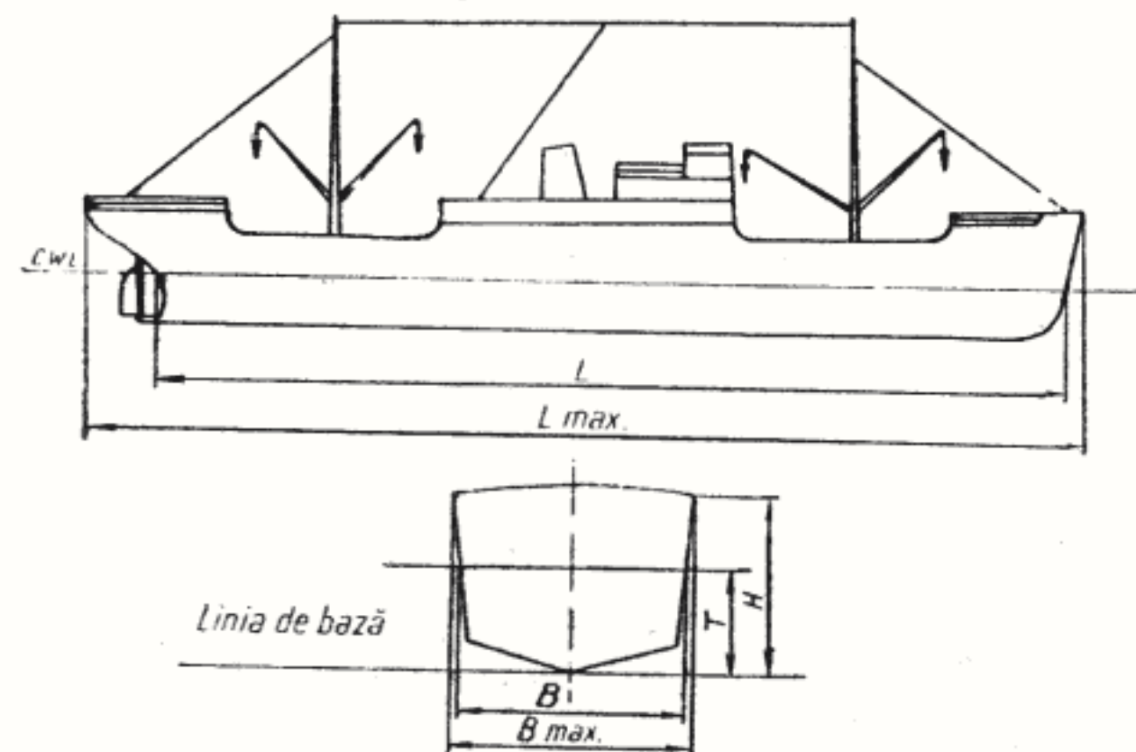
Fig. 9 — Dimensiunile principale ale modelului.
