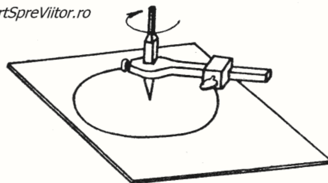
Fig. 3 — Compas pentru tăiat placaj.
