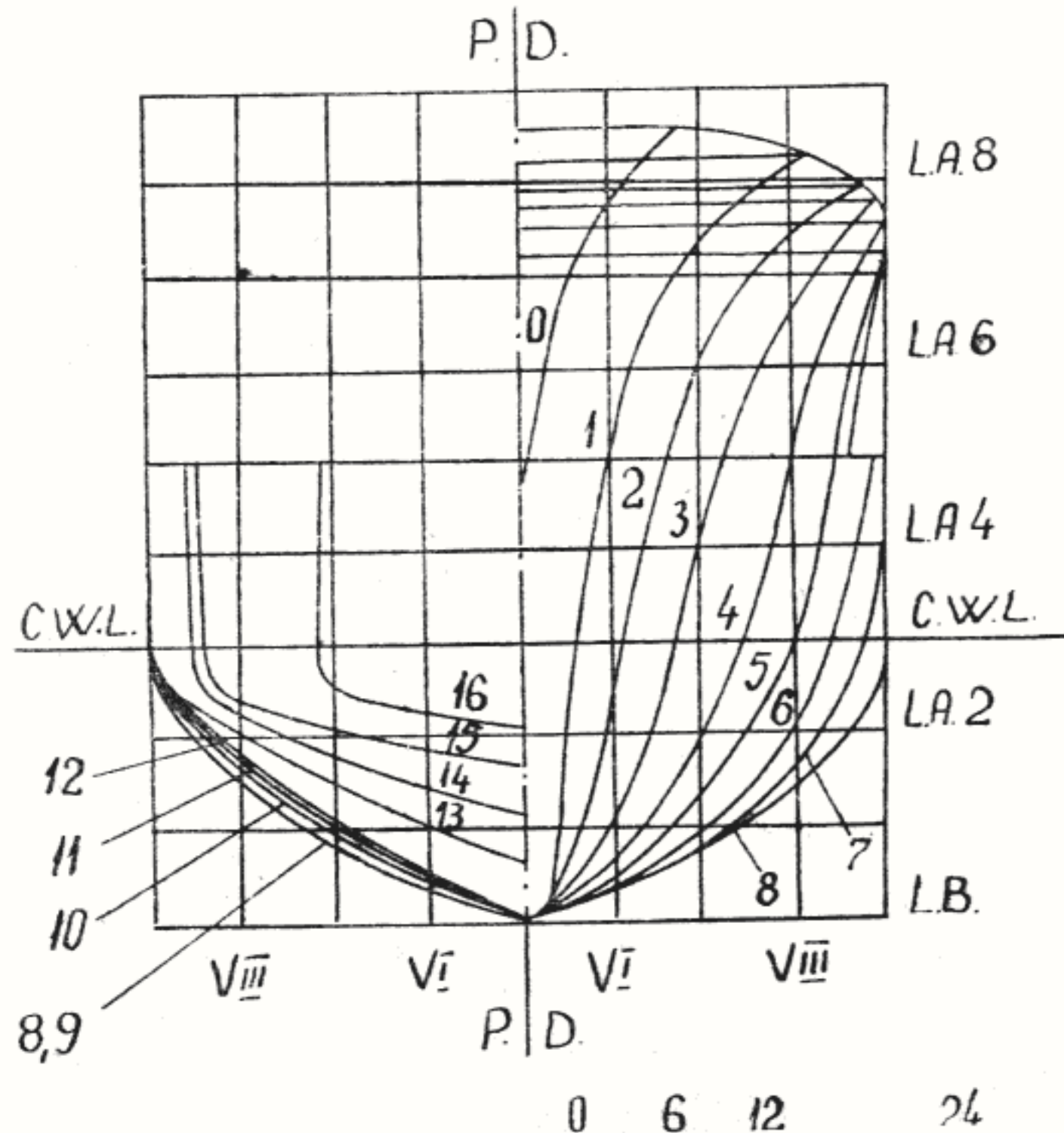
Fig. 68 — Transversalul pe coaste al modelului distrugătorului „Ferdinand”.
