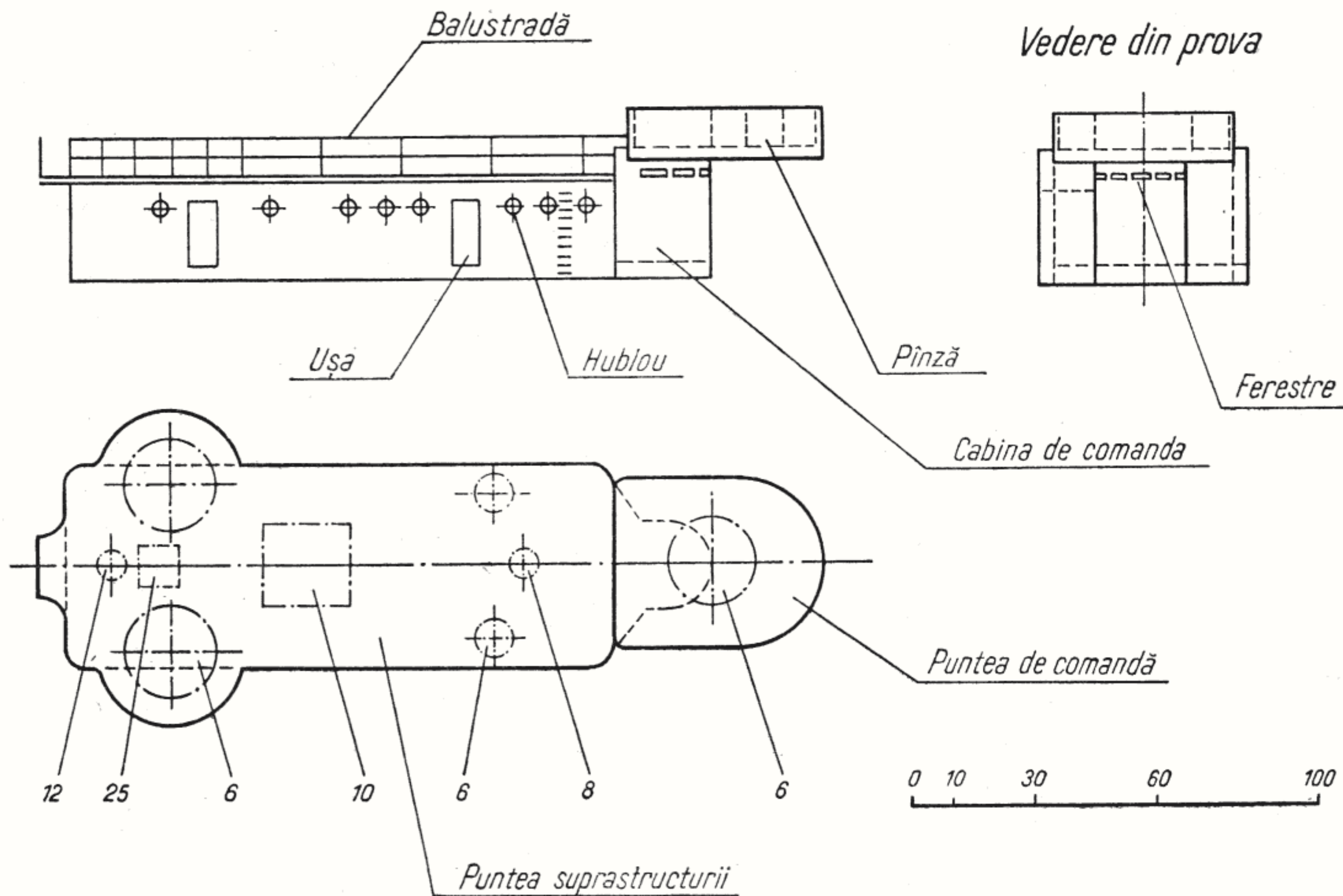
Fig. 76 — Suprastructura modelului monitorului „Alexandru Lahovari“.
