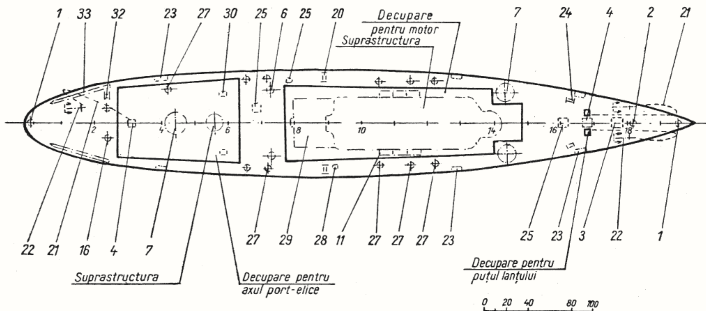
Fig. 75 — Puntea principală pentru modelul monitorului „Alexandru Lahovari“.
