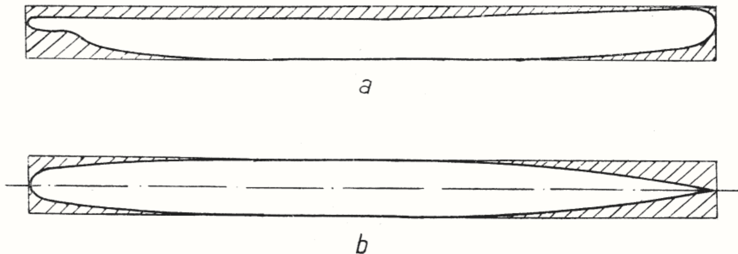
Fig. 64 — a) Trasajul bordajului; b) trasajul punții.
