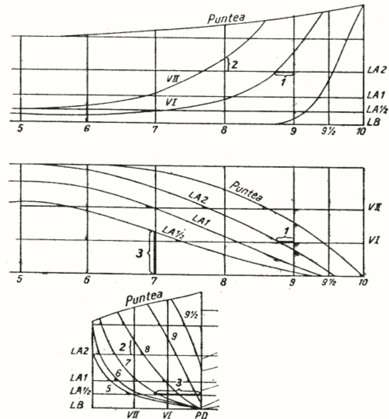
Fig. 20 — Balansarea planului de forme.
