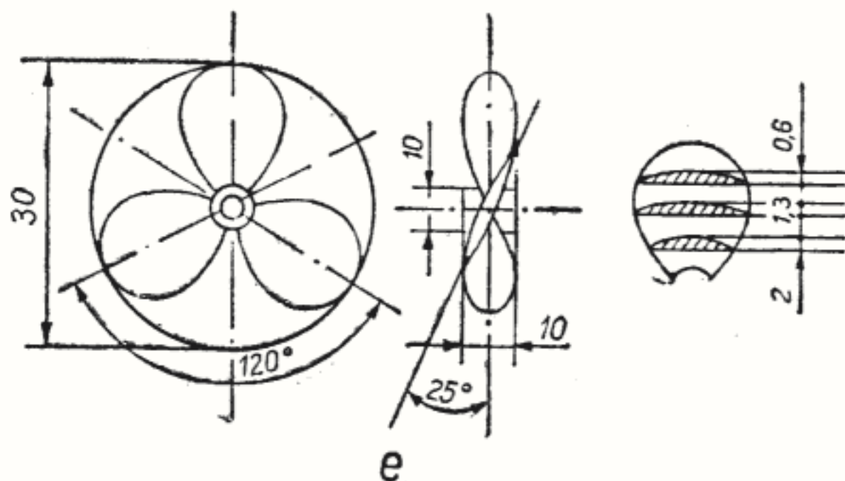
Fig. 84 — Elicea pescadorului „Pălămida“.
