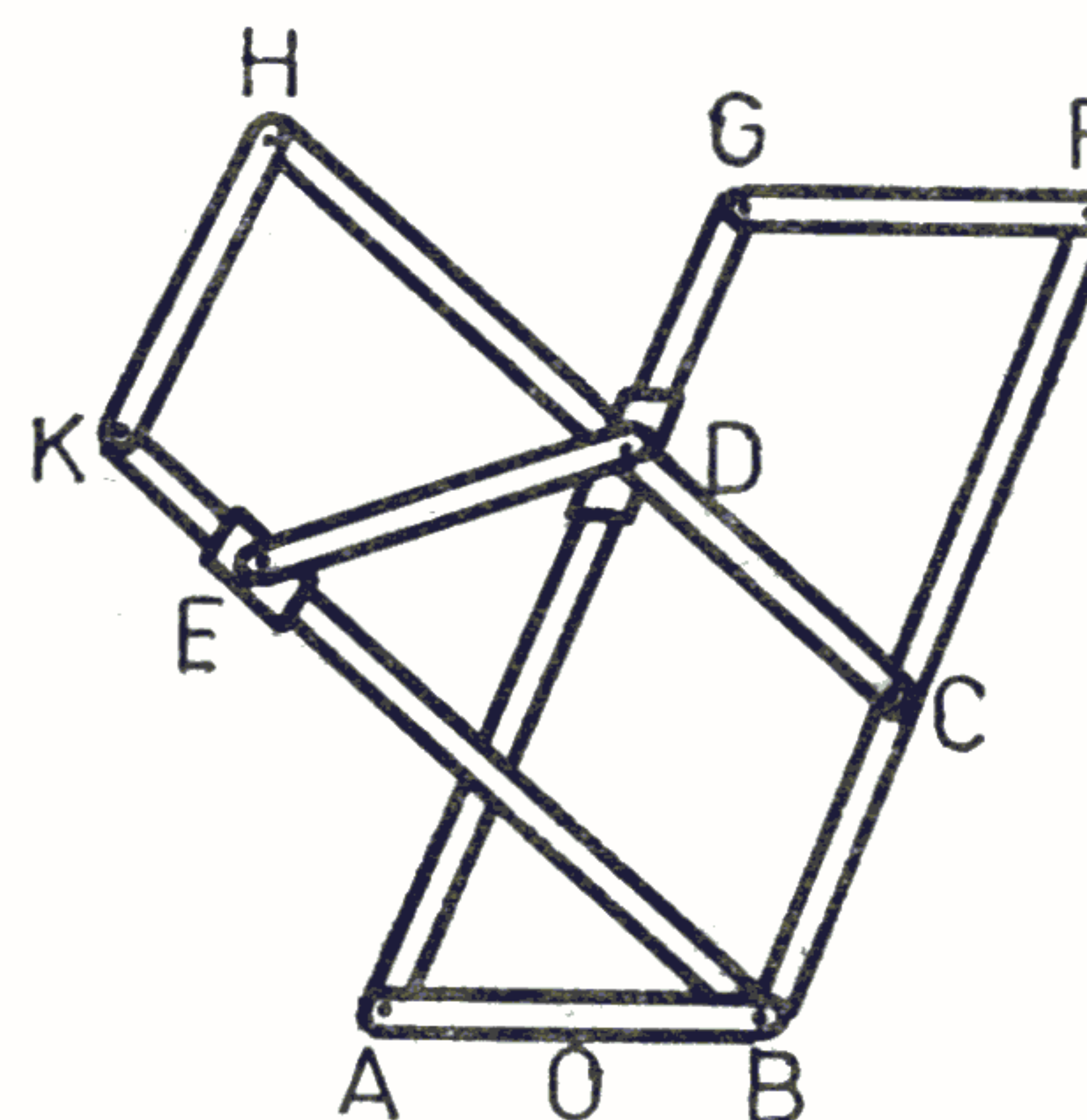
Fig. 18 — Instrument pentru construirea poligoanelor regulate.
