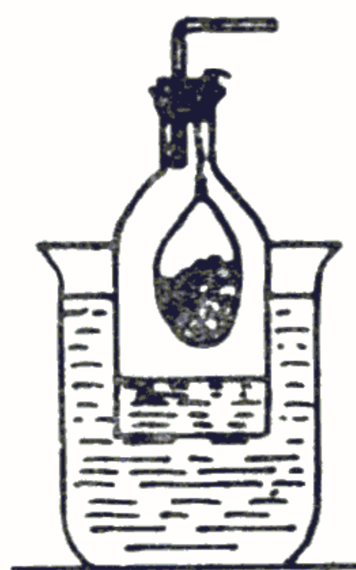
Fig. 26 — Generator de gaze.
