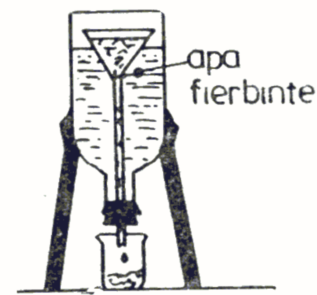
Fig. 28 — Baie pentru încălzirea unei soluții.
