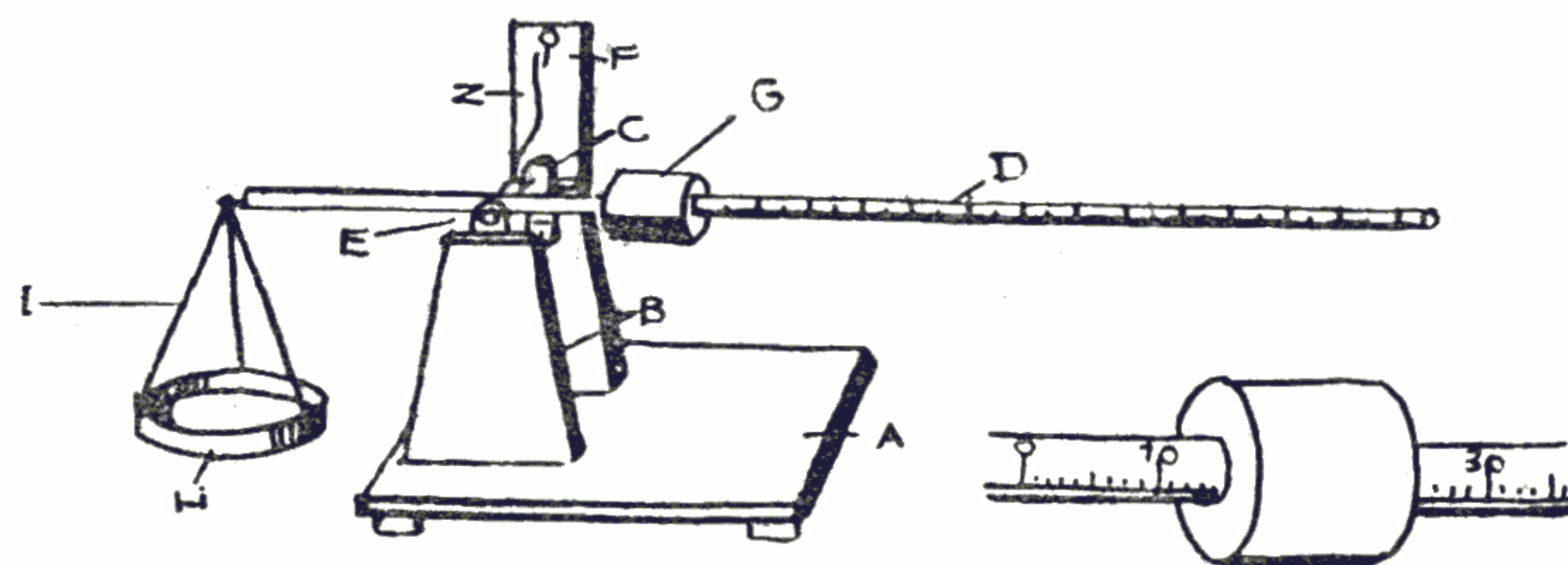
Fig. 16 — Cîntar fără greutăți
