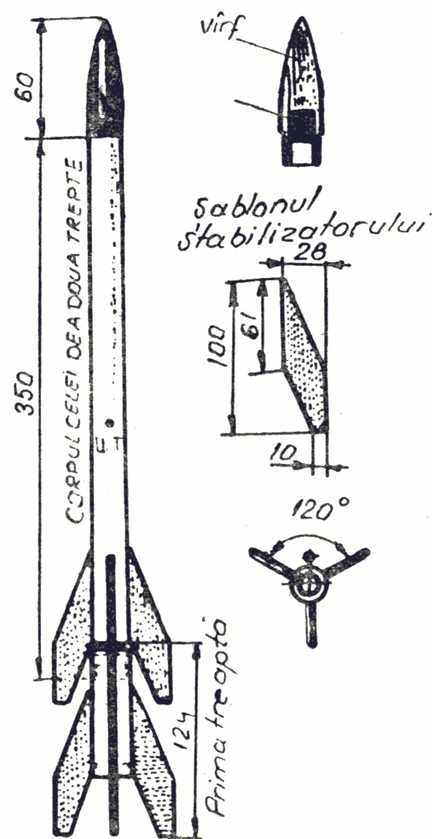
Fig. 32 — Construcția rachetei.
