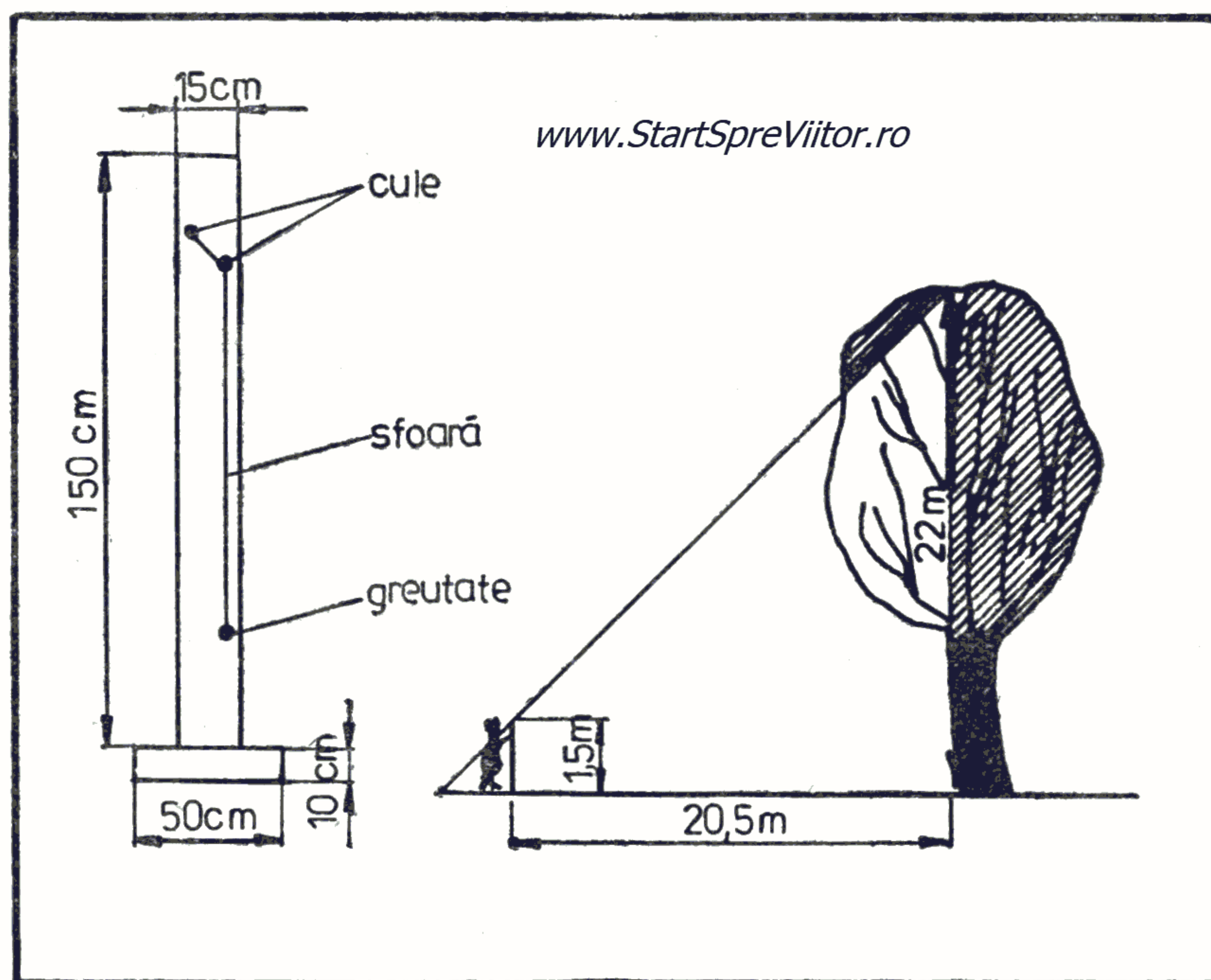
Fig. 15 — Dispozitiv pentru măsurarea înălțimii unor obiecte.
