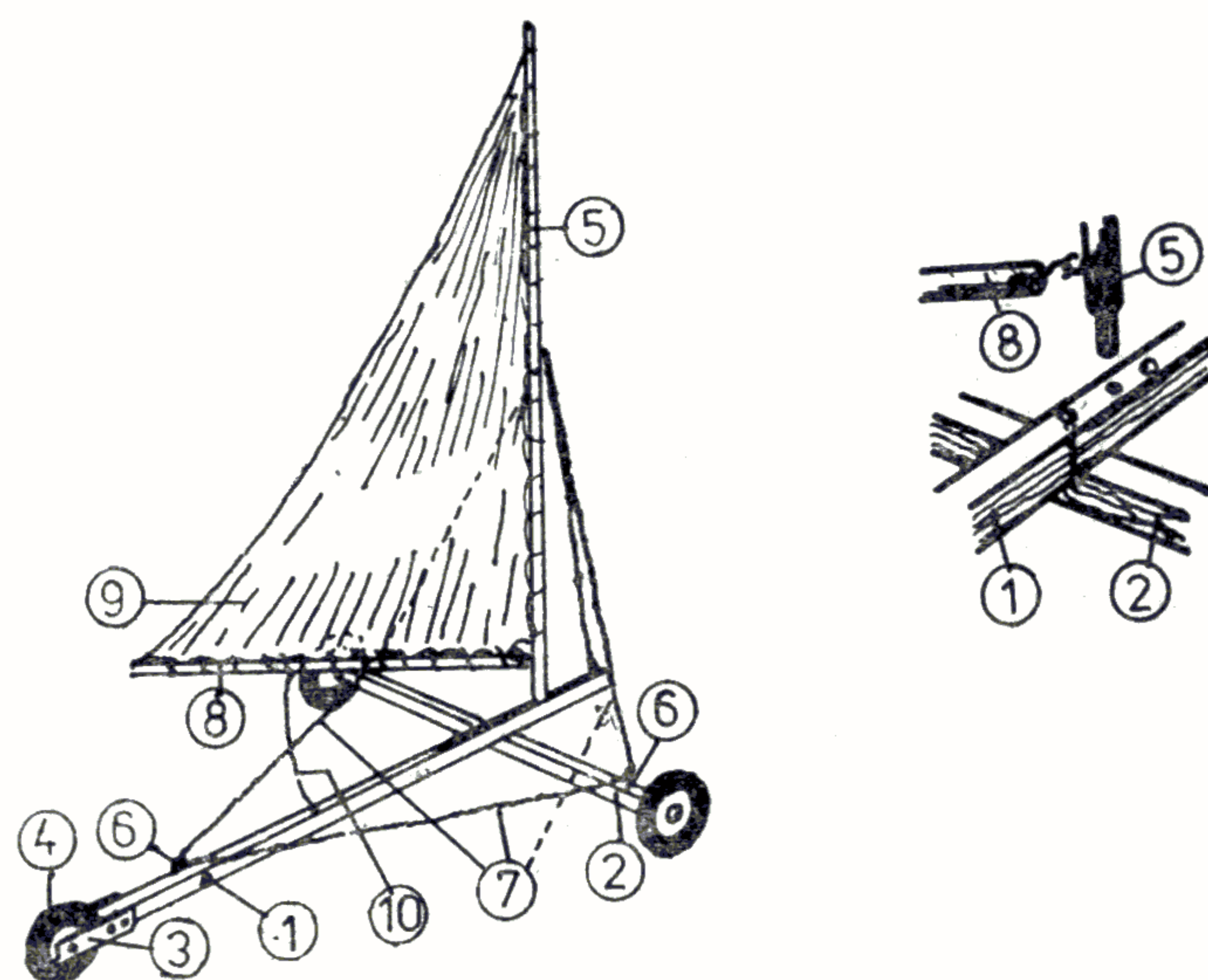
Fig. 33 — Cărucior acționat de forța vântului.
