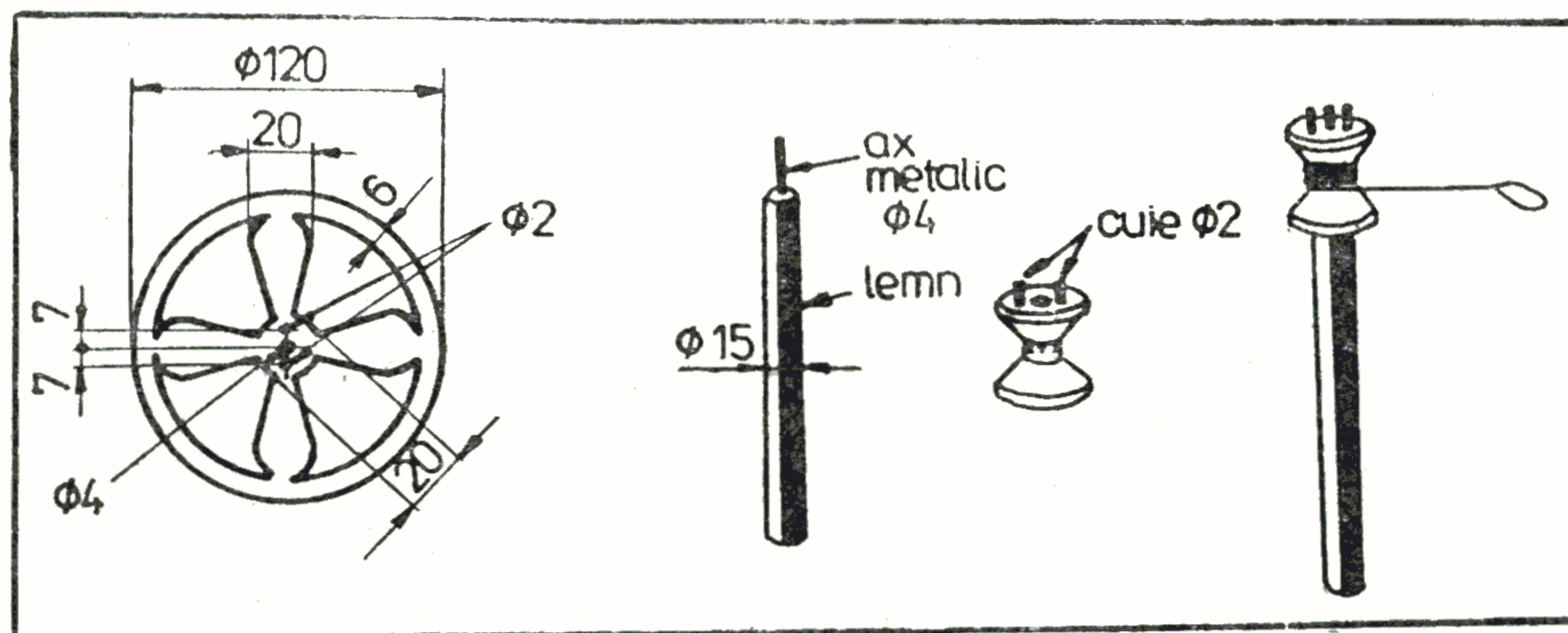
Fig. 29 — Farfuria zburătoare.
