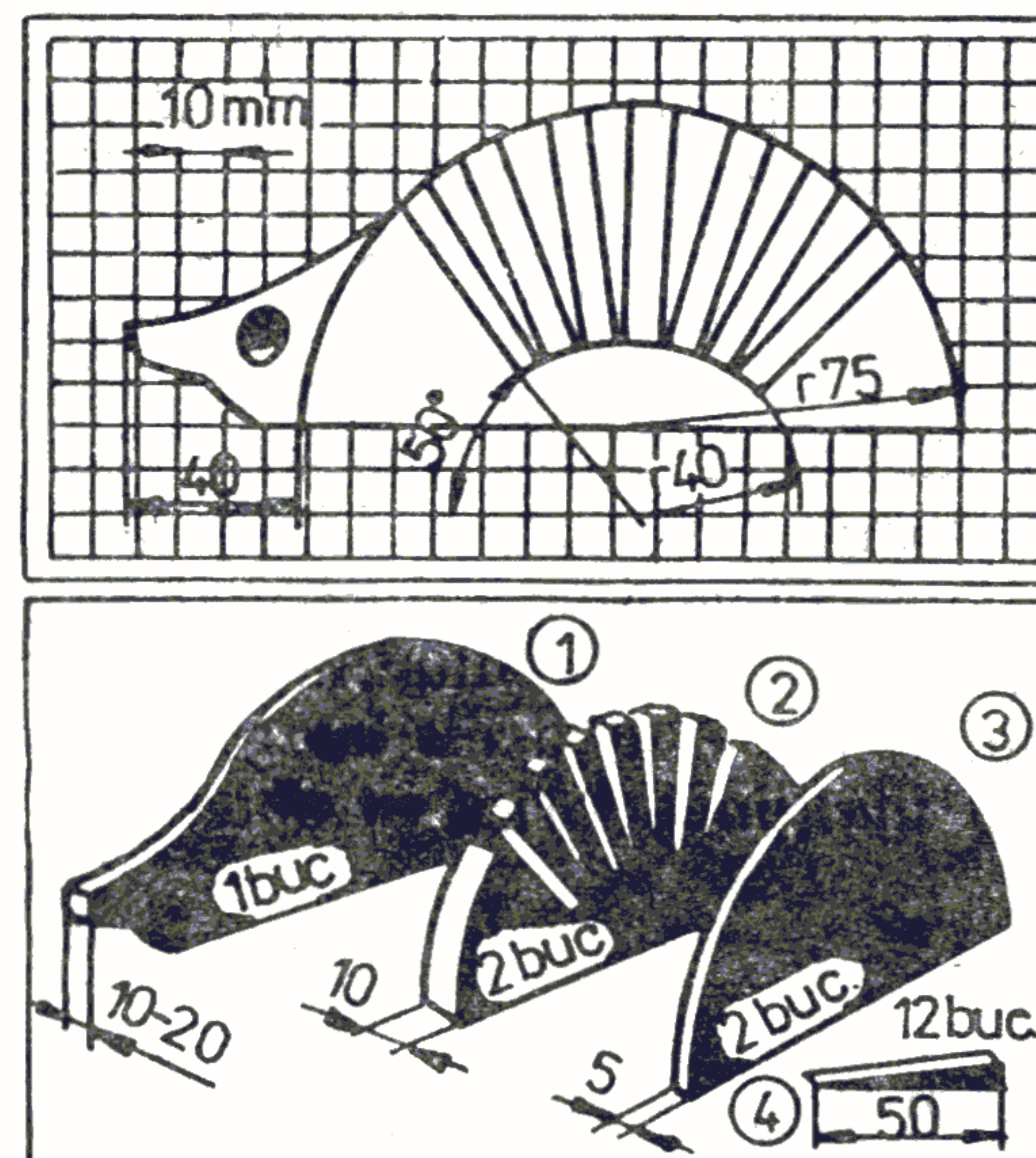
Fig. 17 — Dimensiunile suportului.
