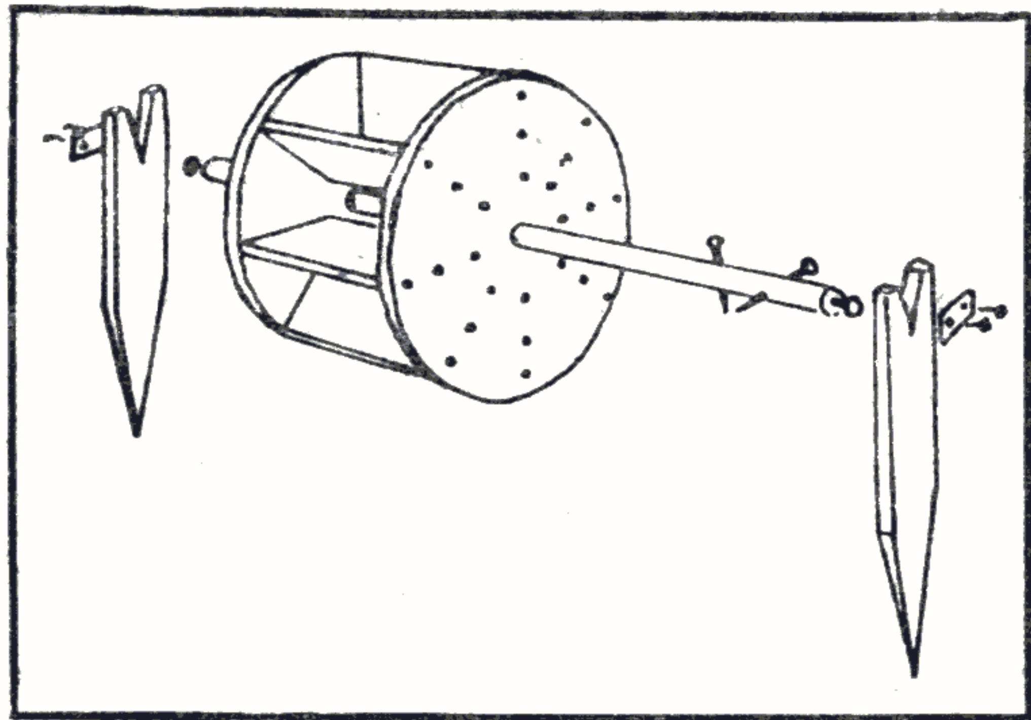
Fig. 36 — Model de roată cu 8 zbaturi.
