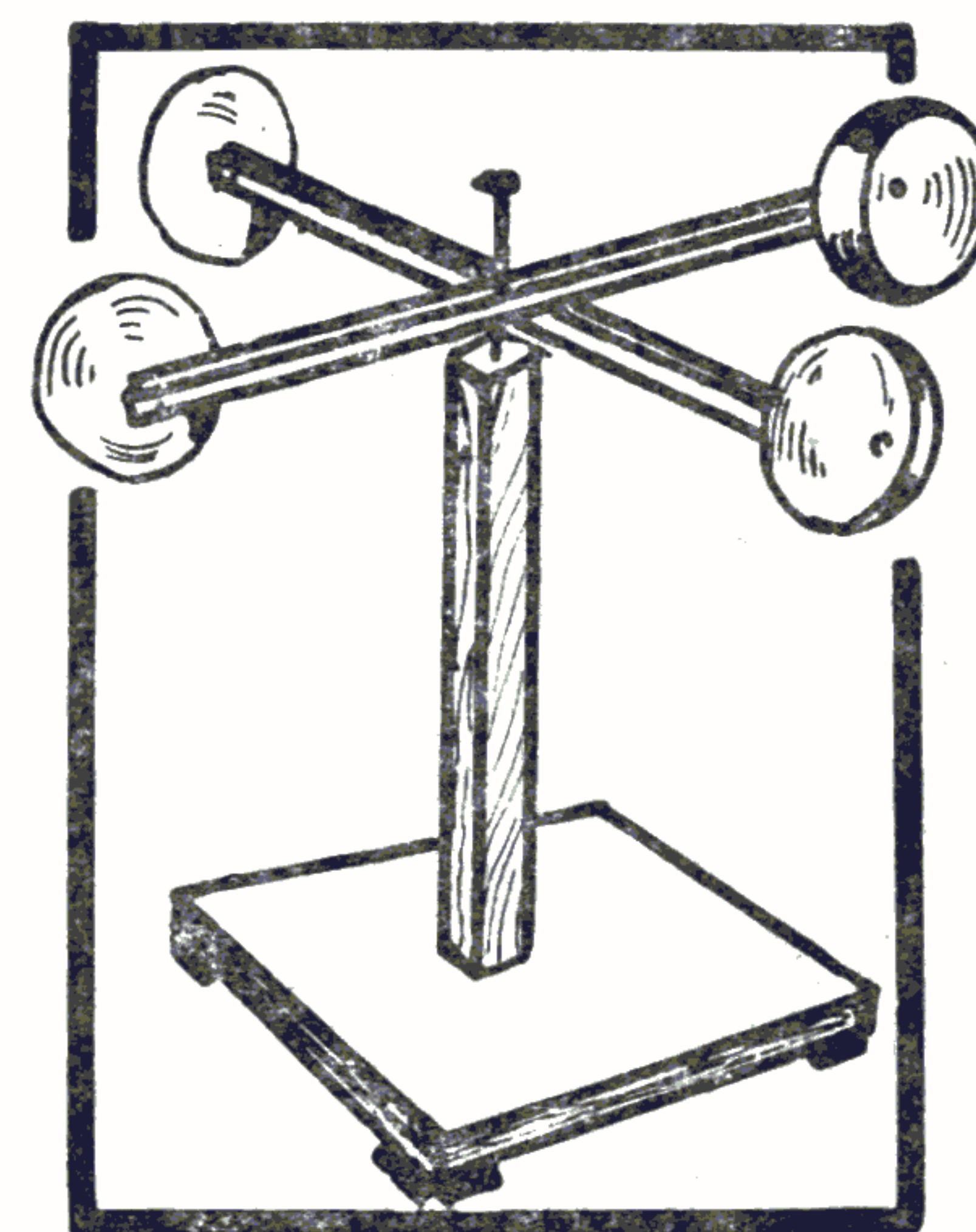
Fig. 11 — Anemometru.
