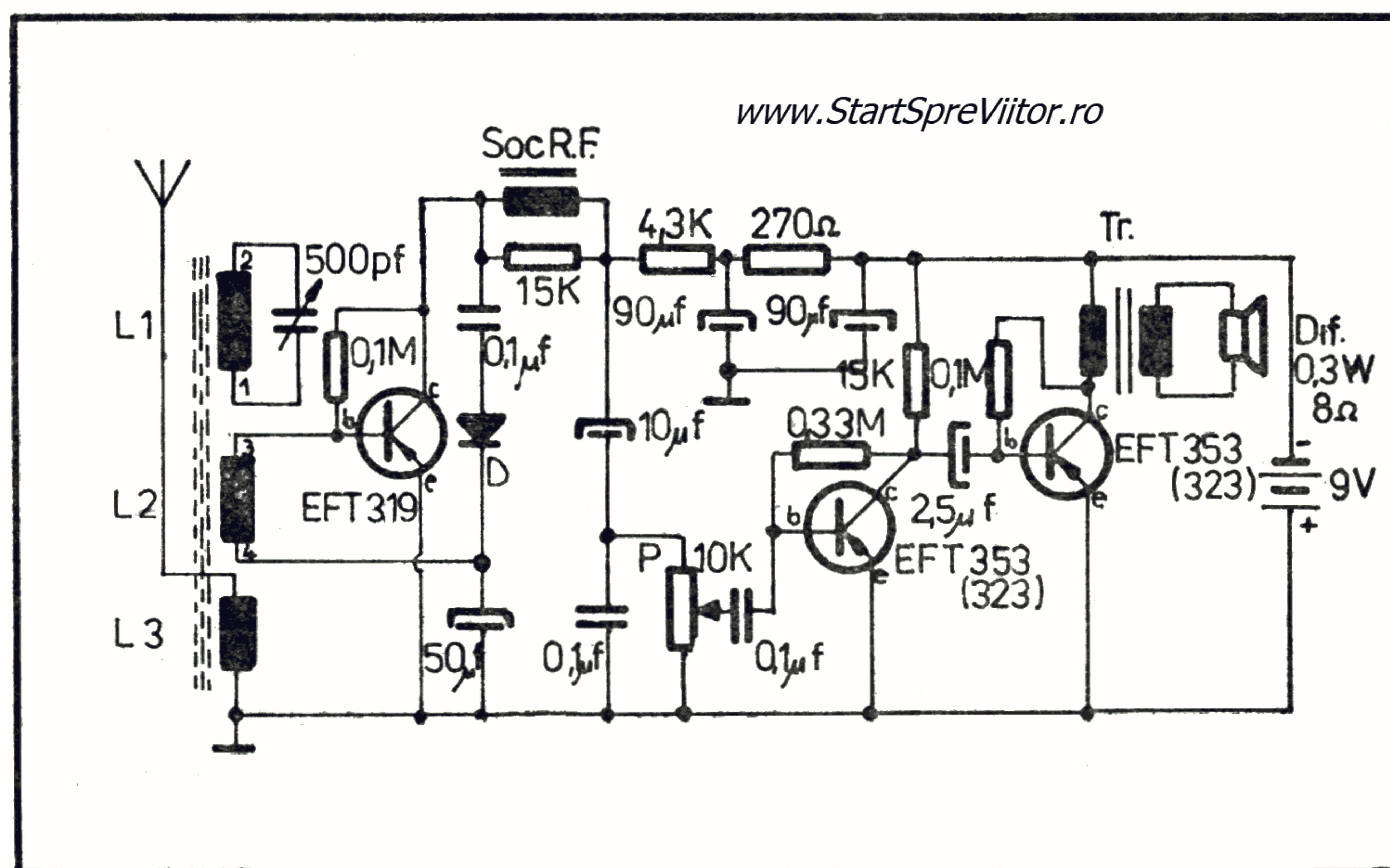
Fig. 42 — Schema receptorului cu 3 tranzistori.
