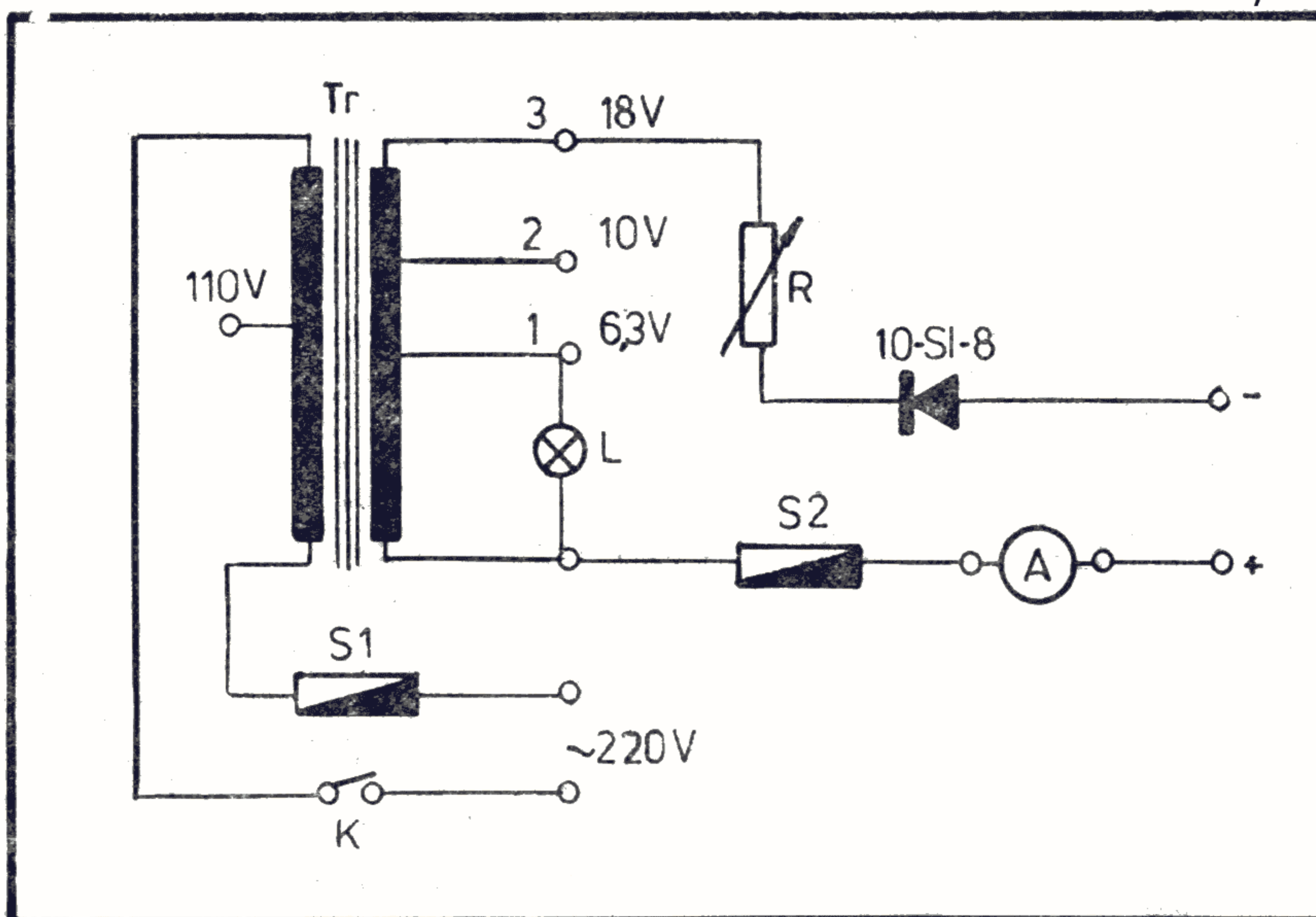
Fig. 39 — Schema redresorului.
