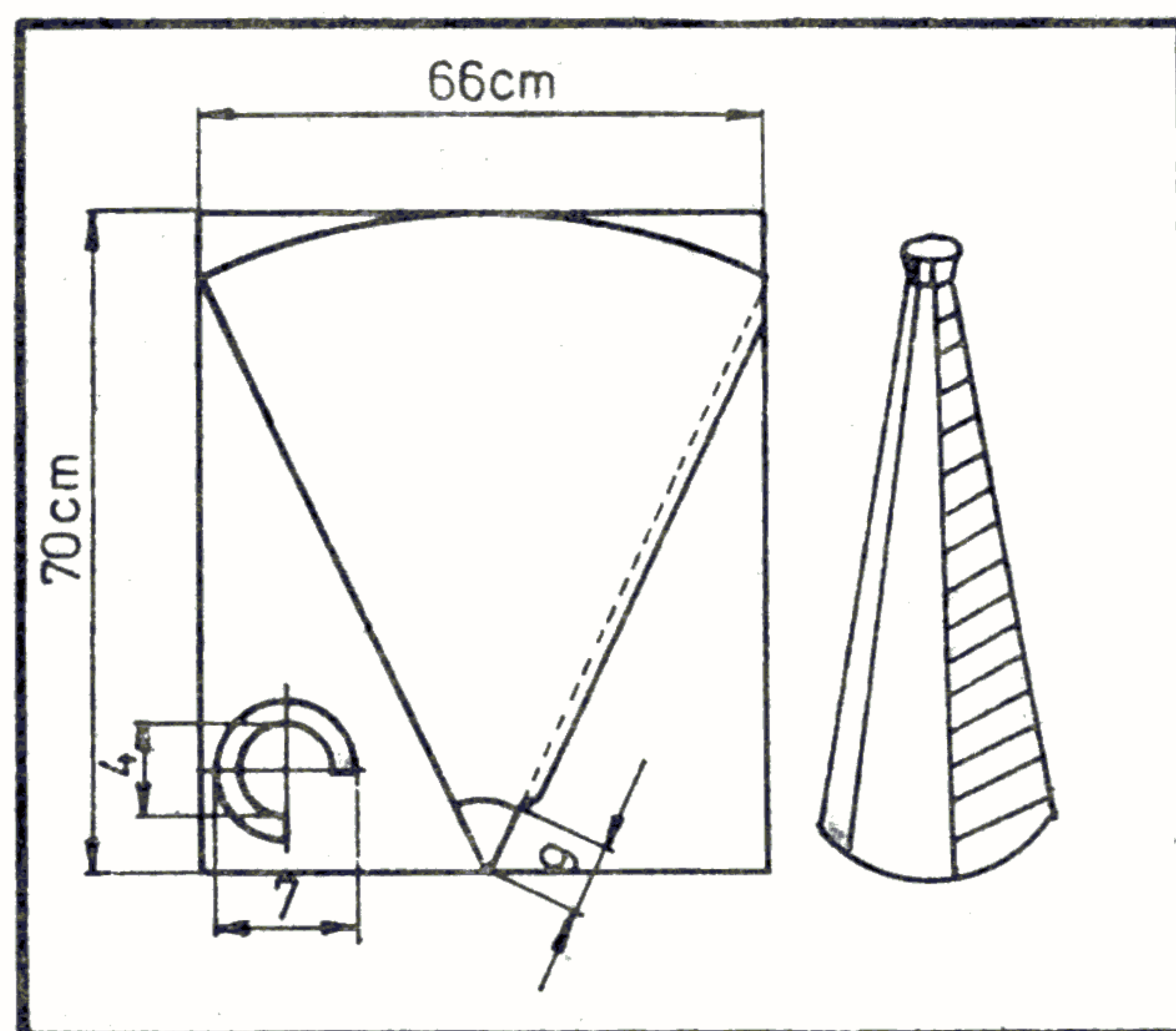
Fig. 5 — Pîlnie portavoce.
