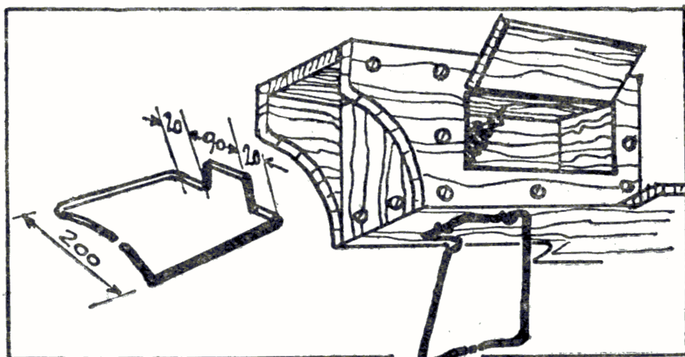
Fig. 22 — Fixarea reazemului basculant.
