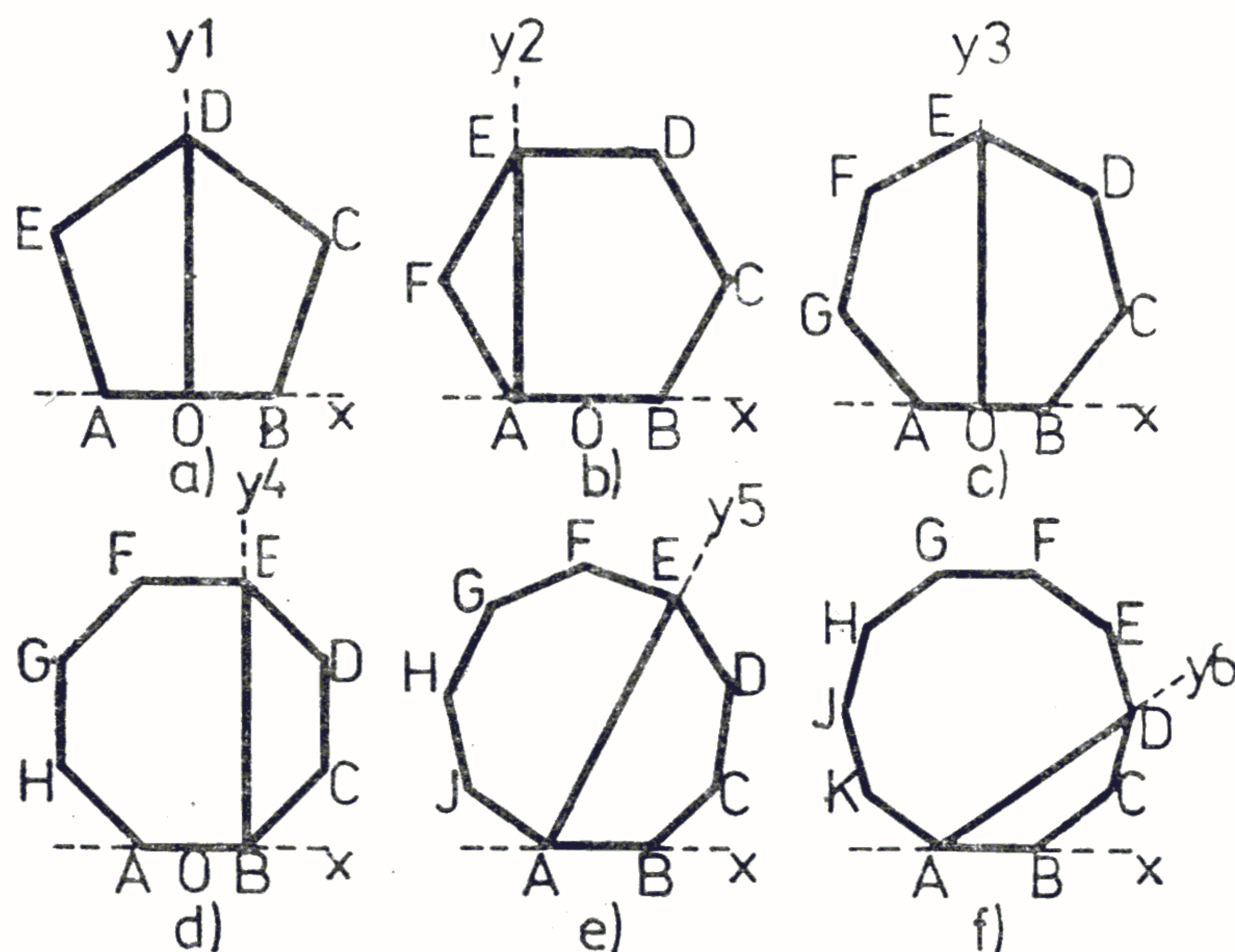
Fig. 19 — Construirea poligoanelor regulate.
