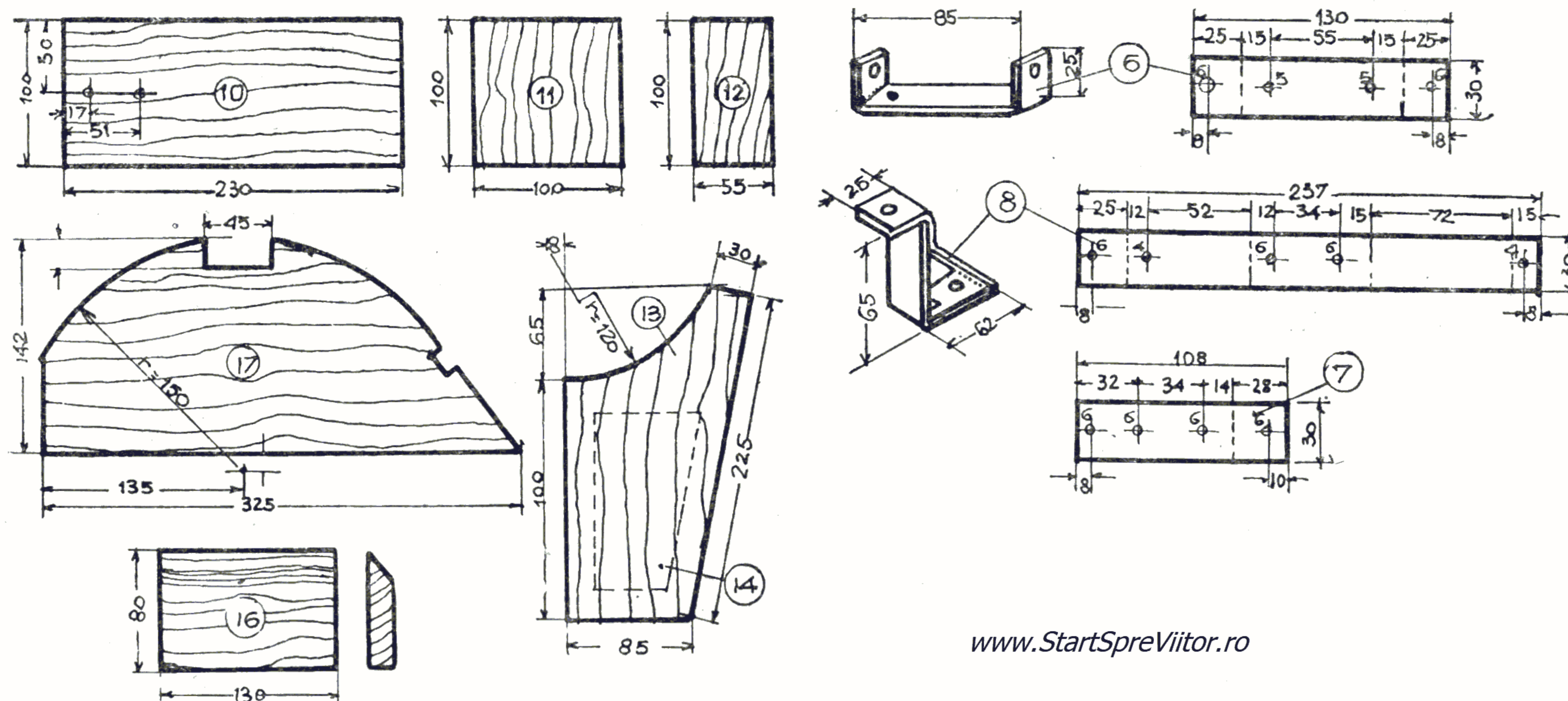
Fig. 20 b — Trotineta „Super“ — detalii constructive.
