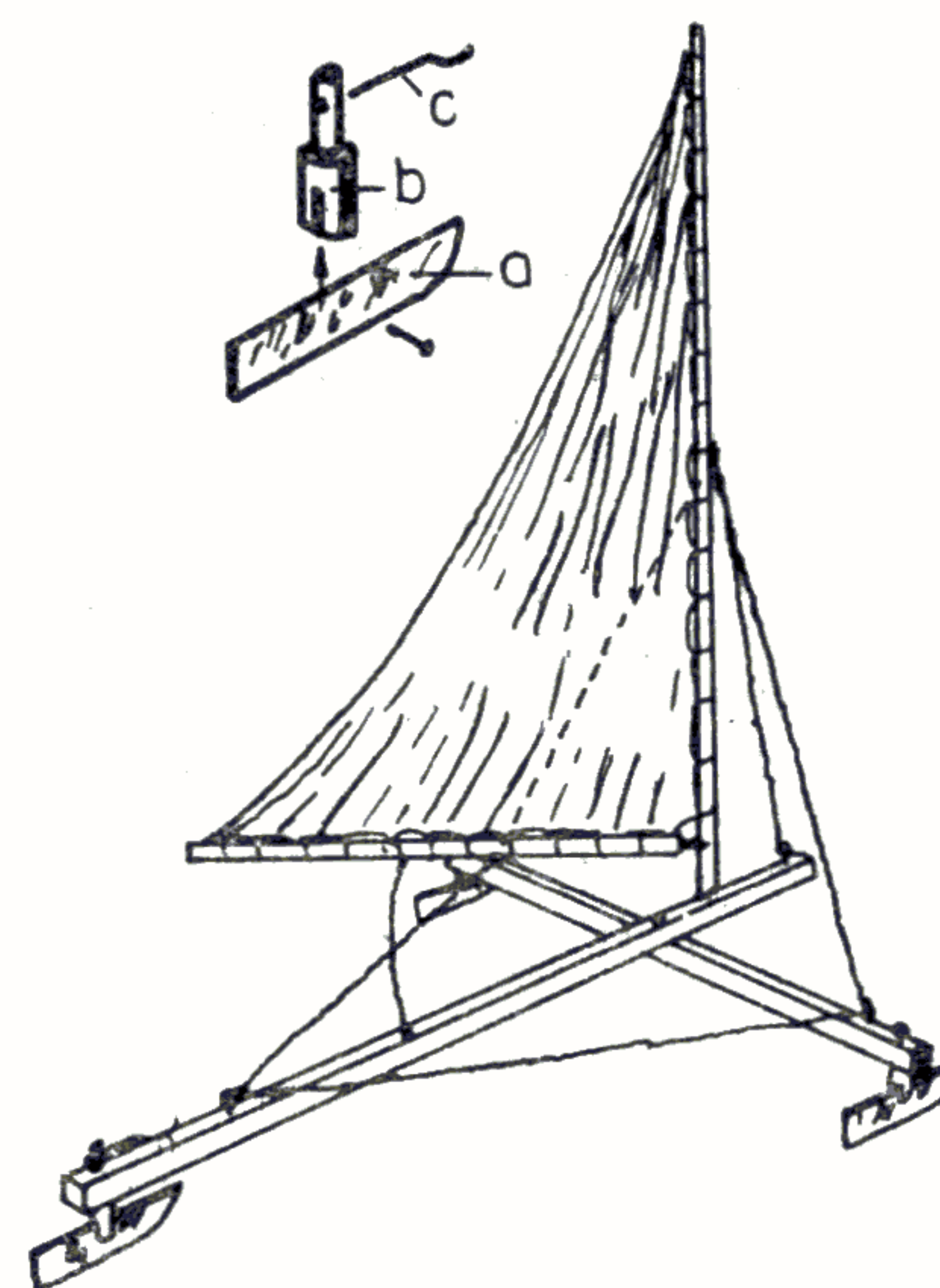
Fig. 34 — Sanie acționată de forța vântului
