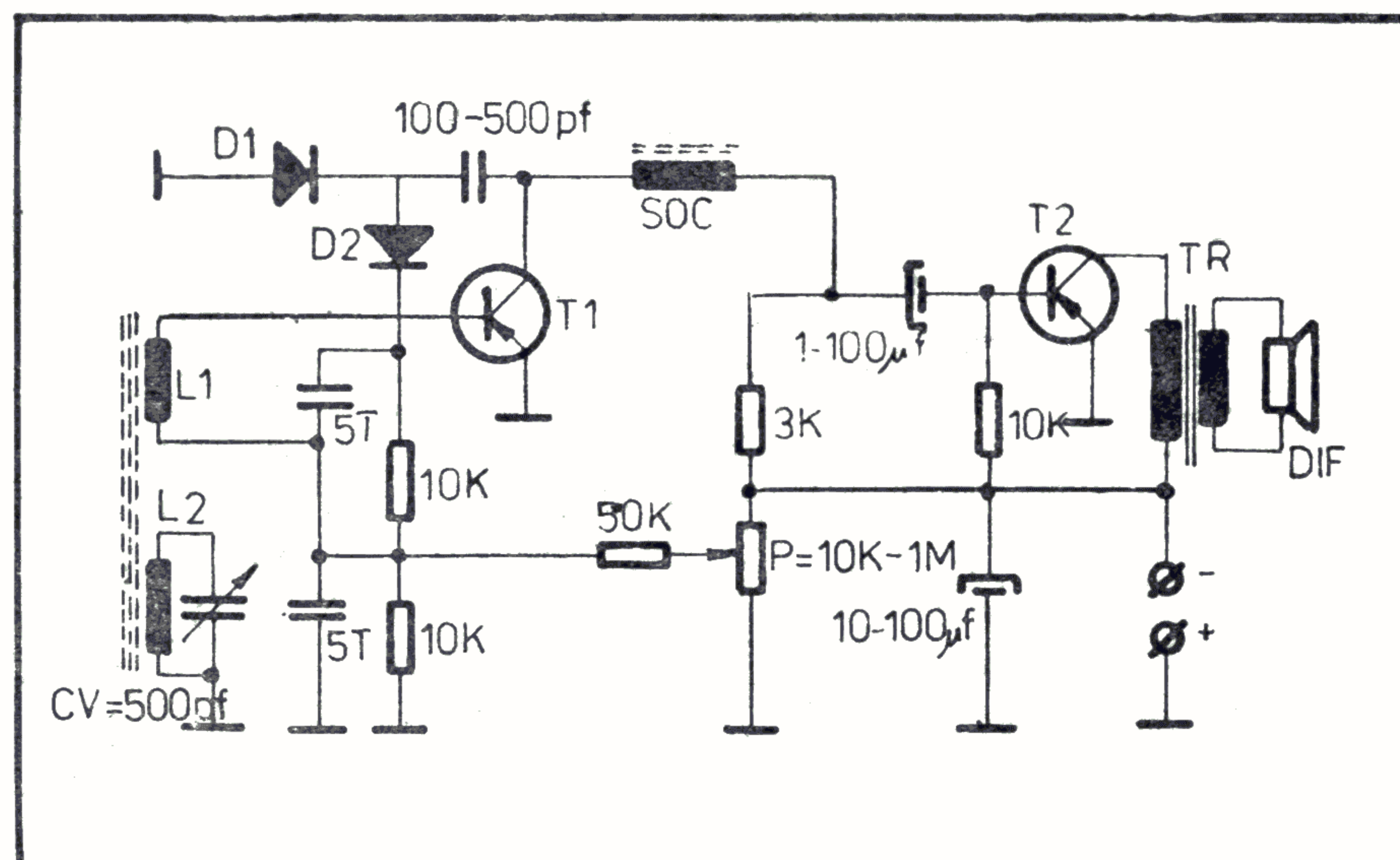
Fig. 41 — Schema receptorului cu 2 tranzistori.
