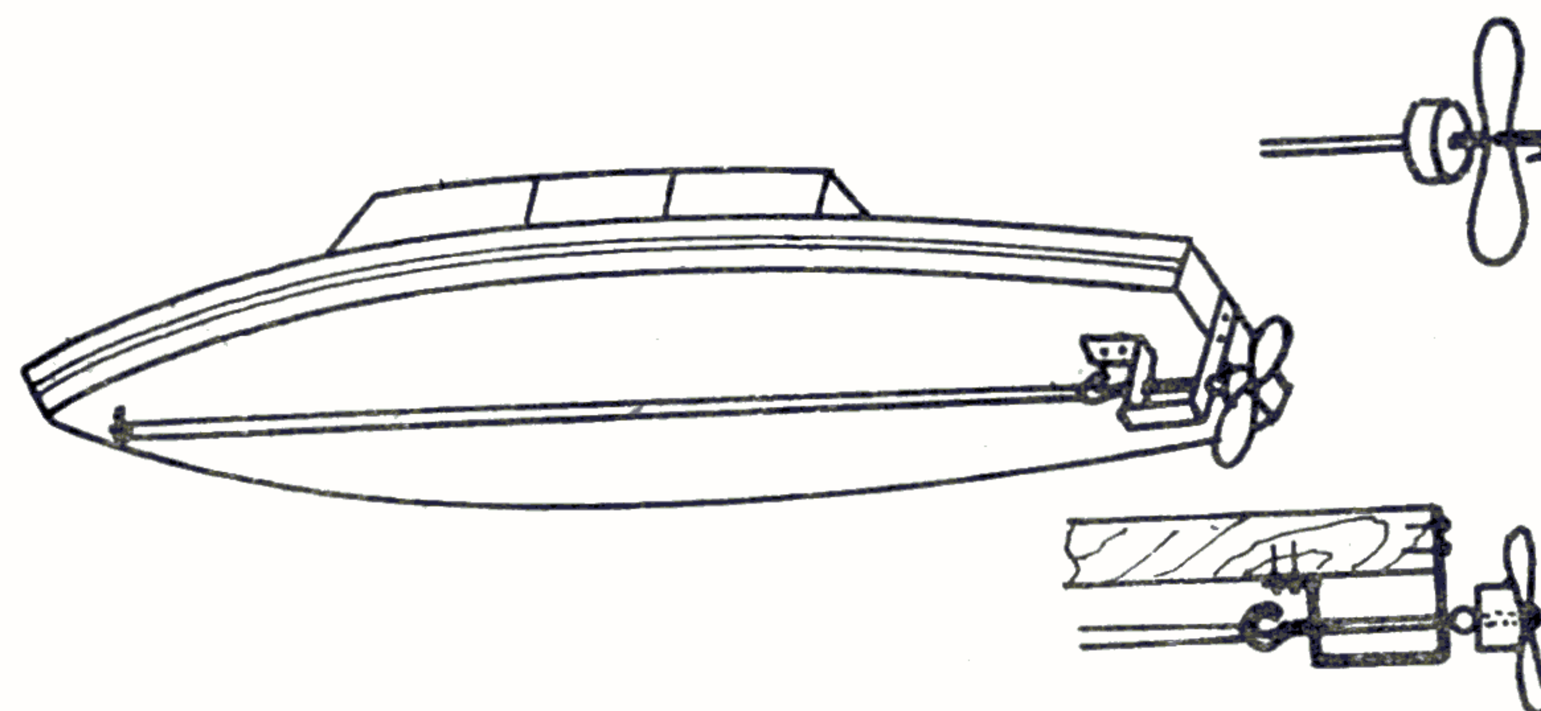
Fig. 14 — Micronavă cu elice.
