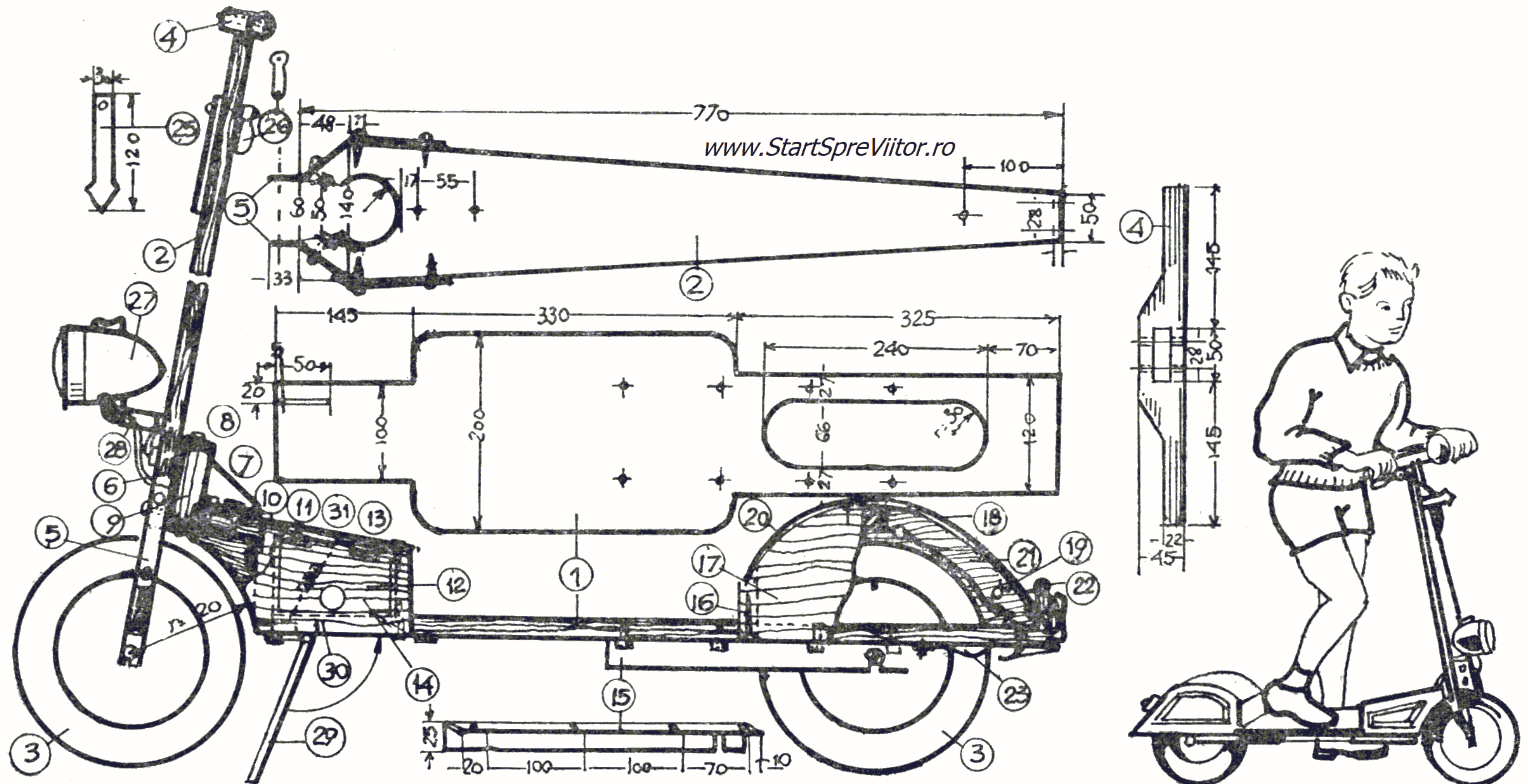
Fig. 20 a — Trotineta „Super“ — vedere laterală.
