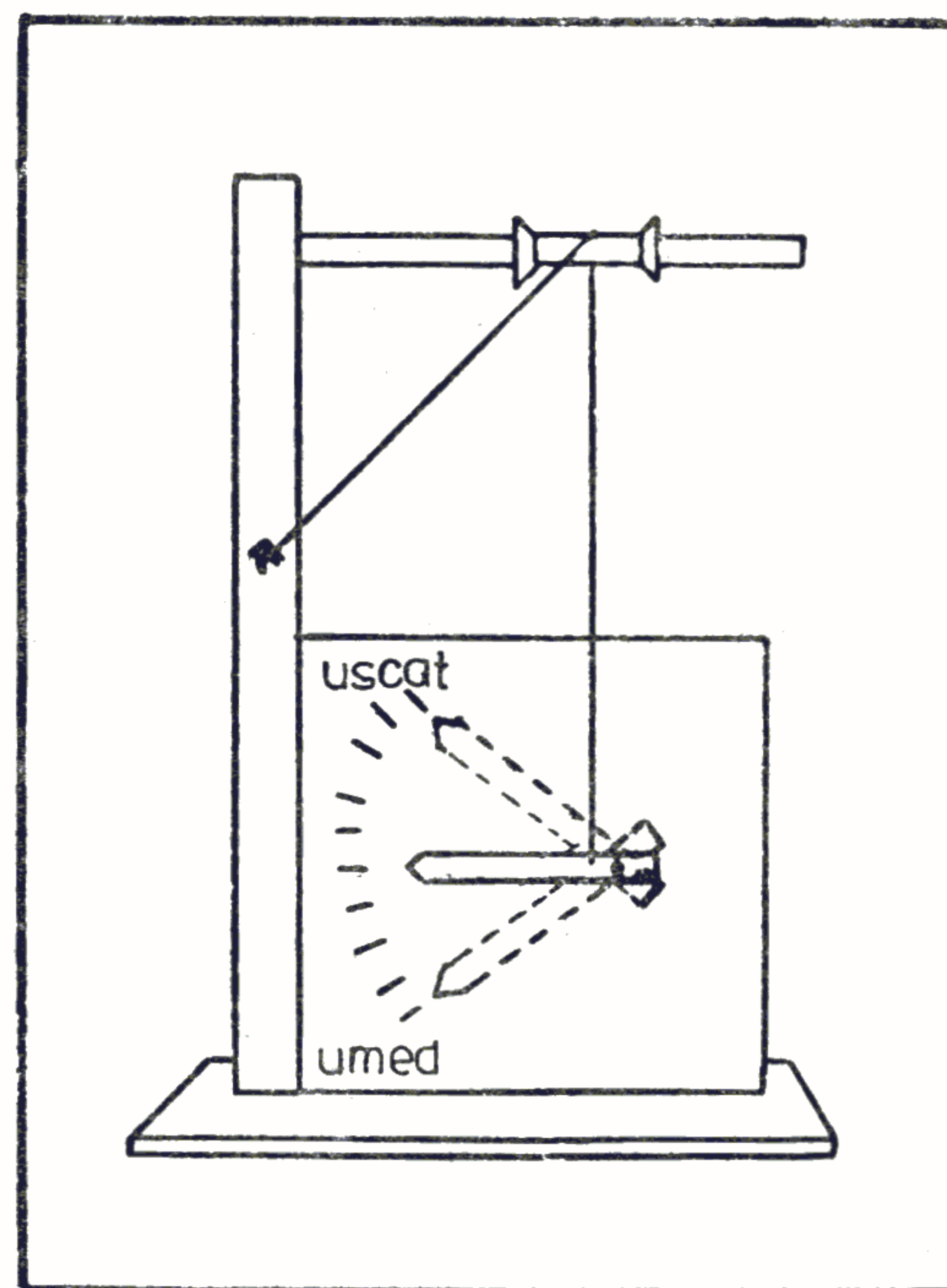
Fig. 12 — Construcția higrometrului.
