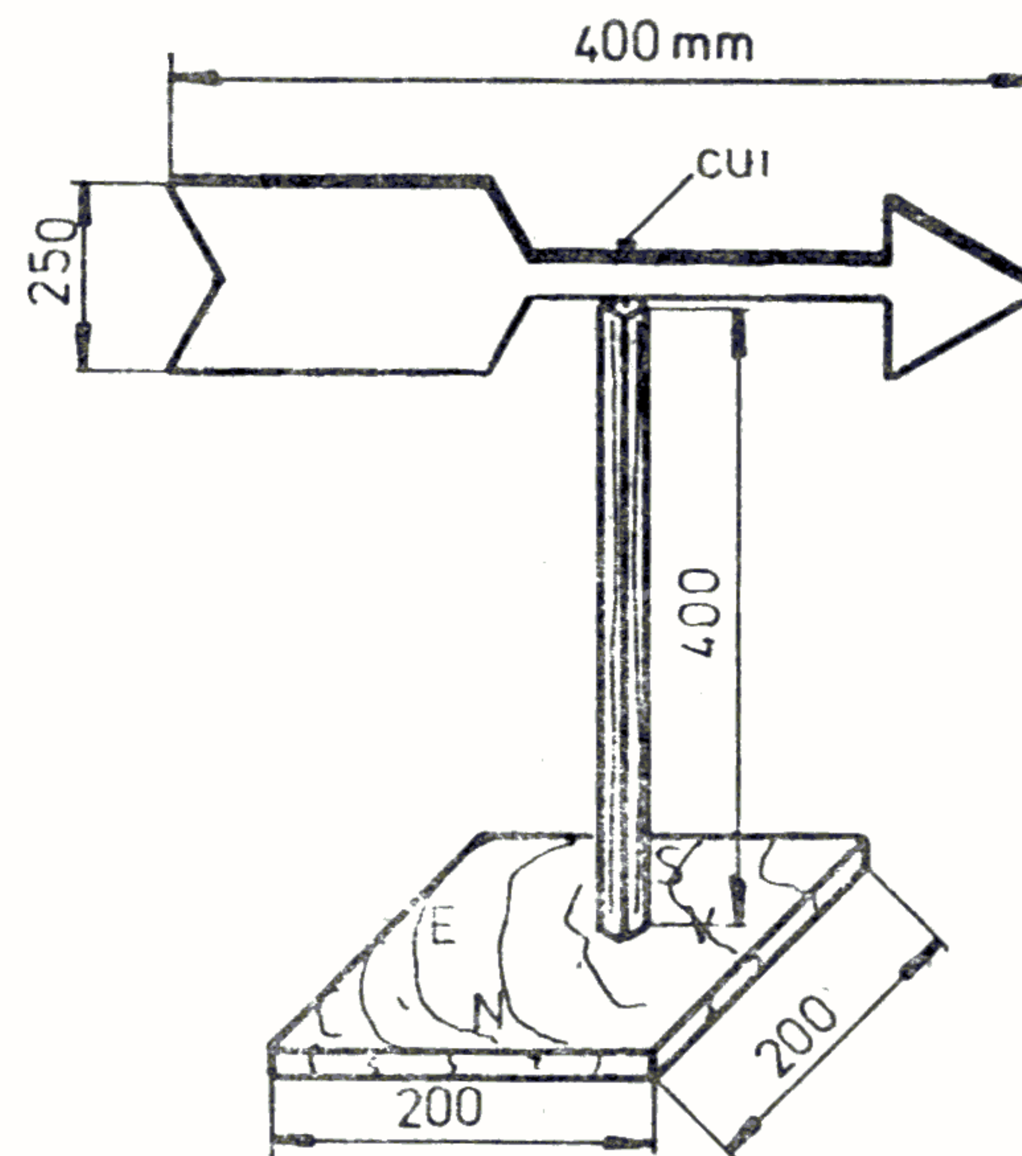
Fig. 9 — Girueta.
