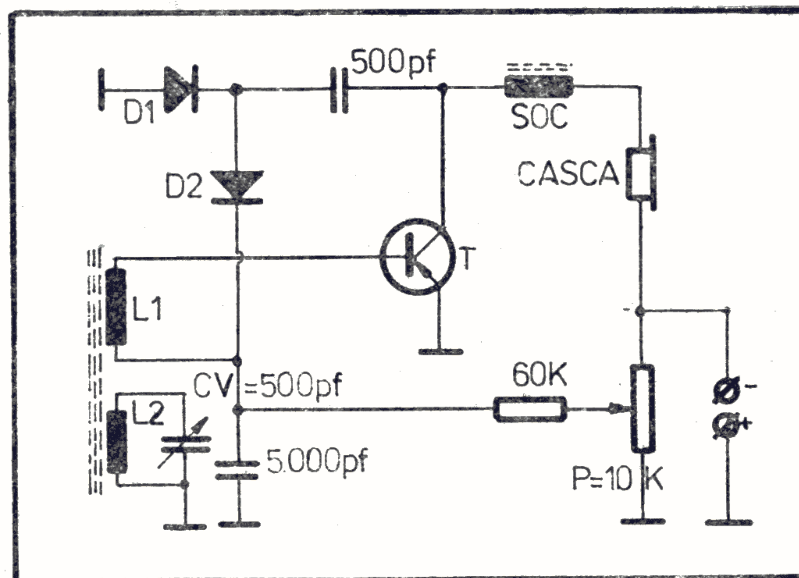
Fig. 40 — Schema receptorului cu 1 tranzistor.
