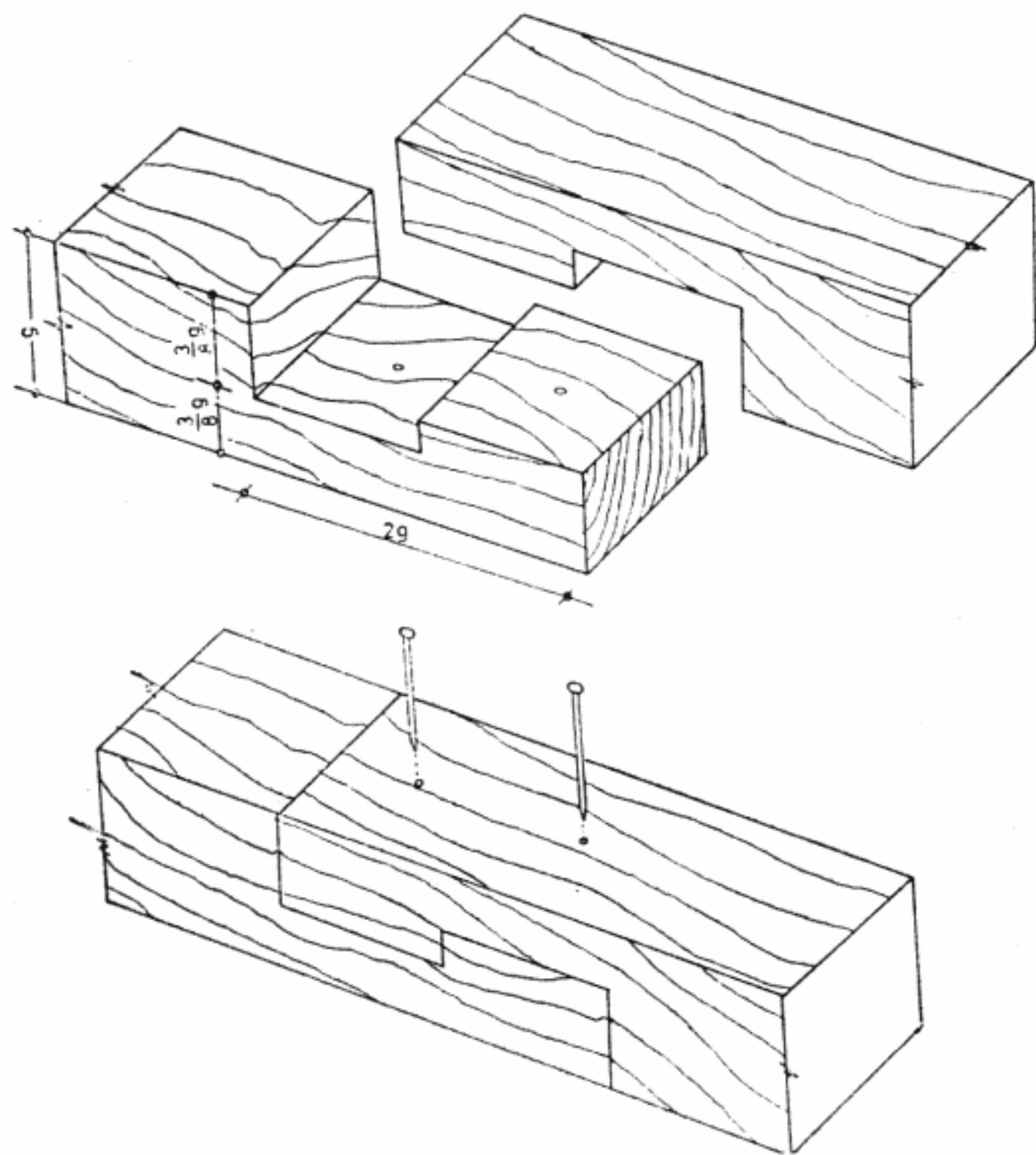
Fig. 12. — Innădire cu prag simplu
