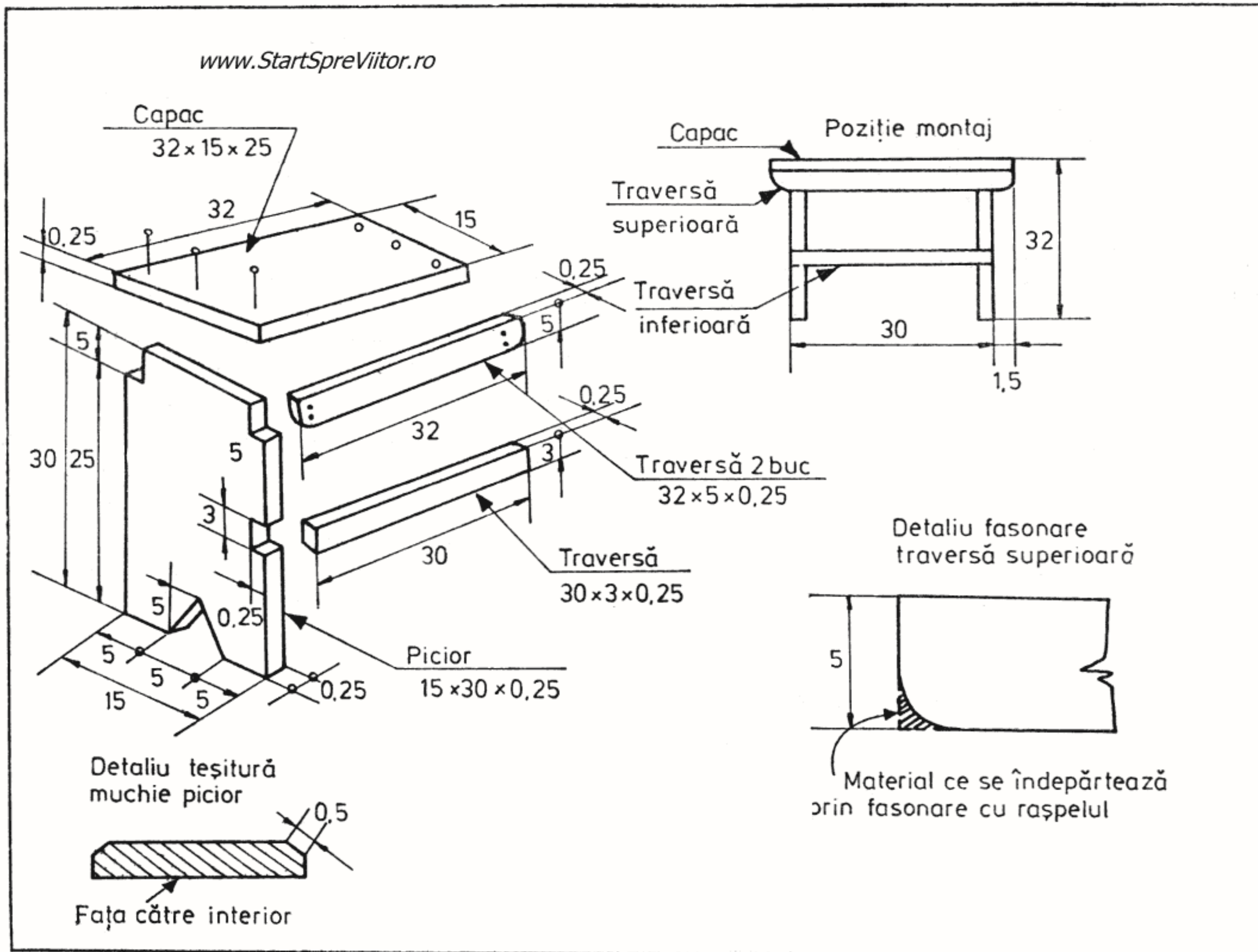
Fig. 37 — Scăunel de lemn
