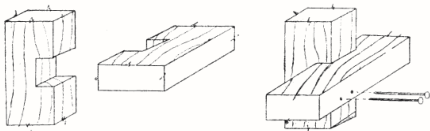
Fig. 4 — Chertare format T pentru încrucișări
