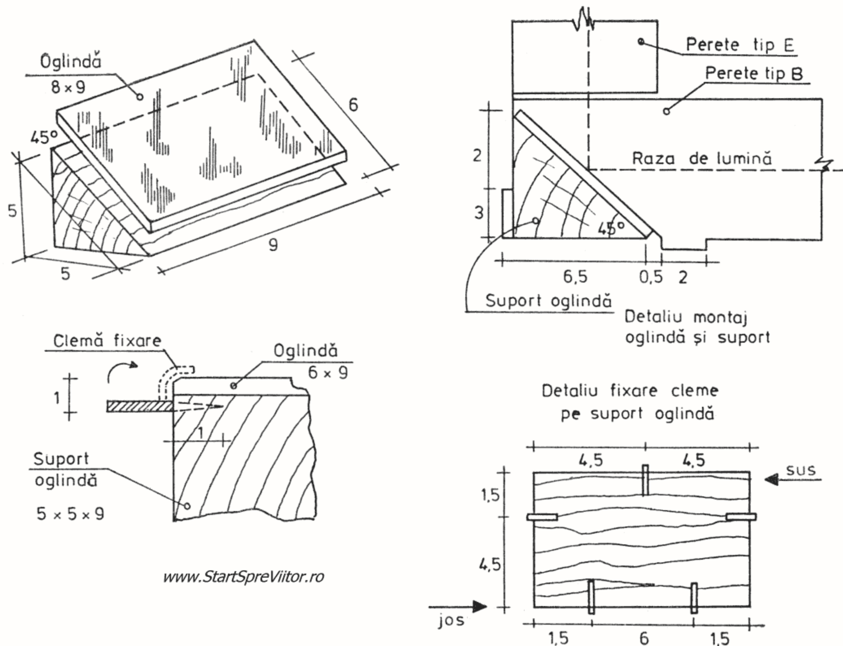
Fig. 28 — Suportul cu oglindă
