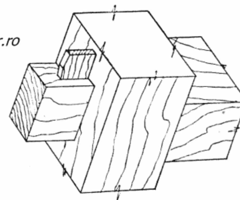
Fig. 13 — Îmbinare demontabilă
