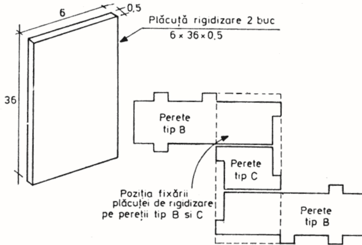
Fig. 29 — Montarea plăcuței de rigidizare
