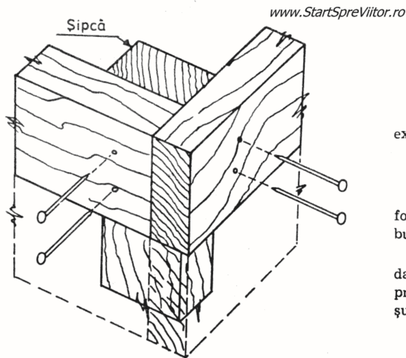
Fig. 10 — Îmbinare de colț cu șipcă interioară
