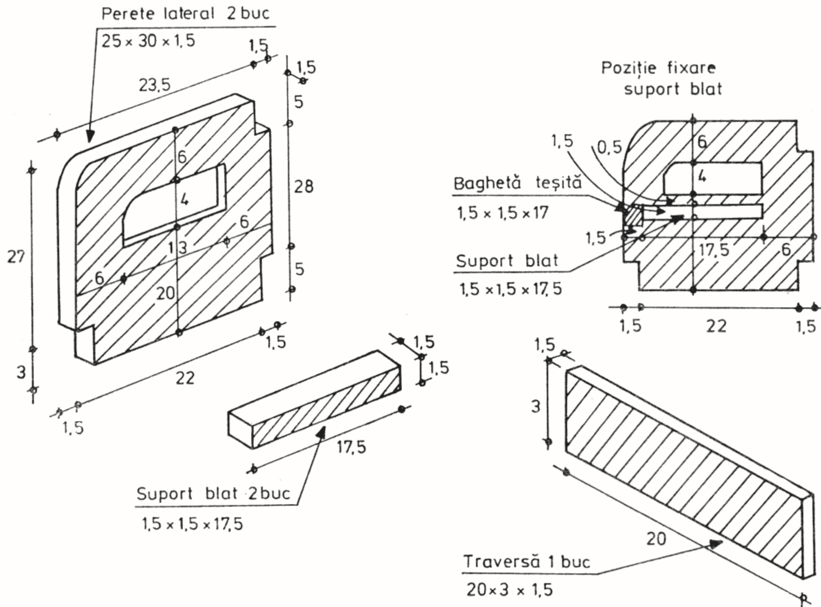
Fig. 35 — Scăunel
