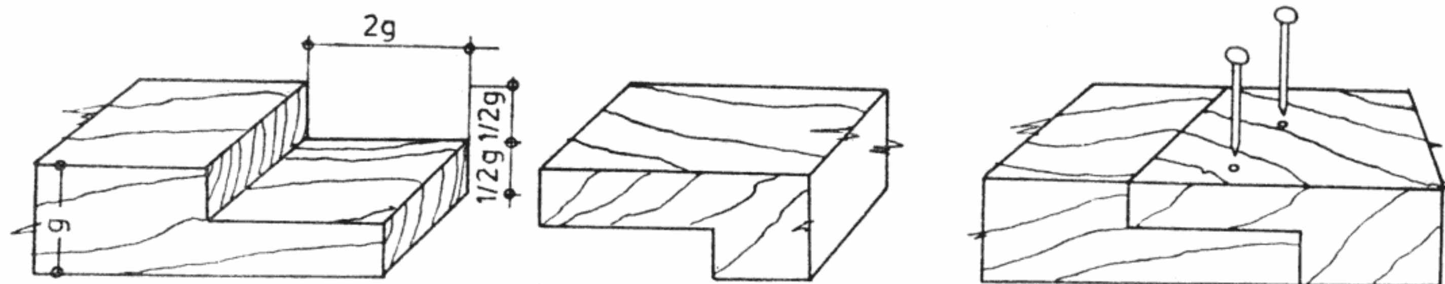
Fig. 1 — Chertare pentru înădăire
