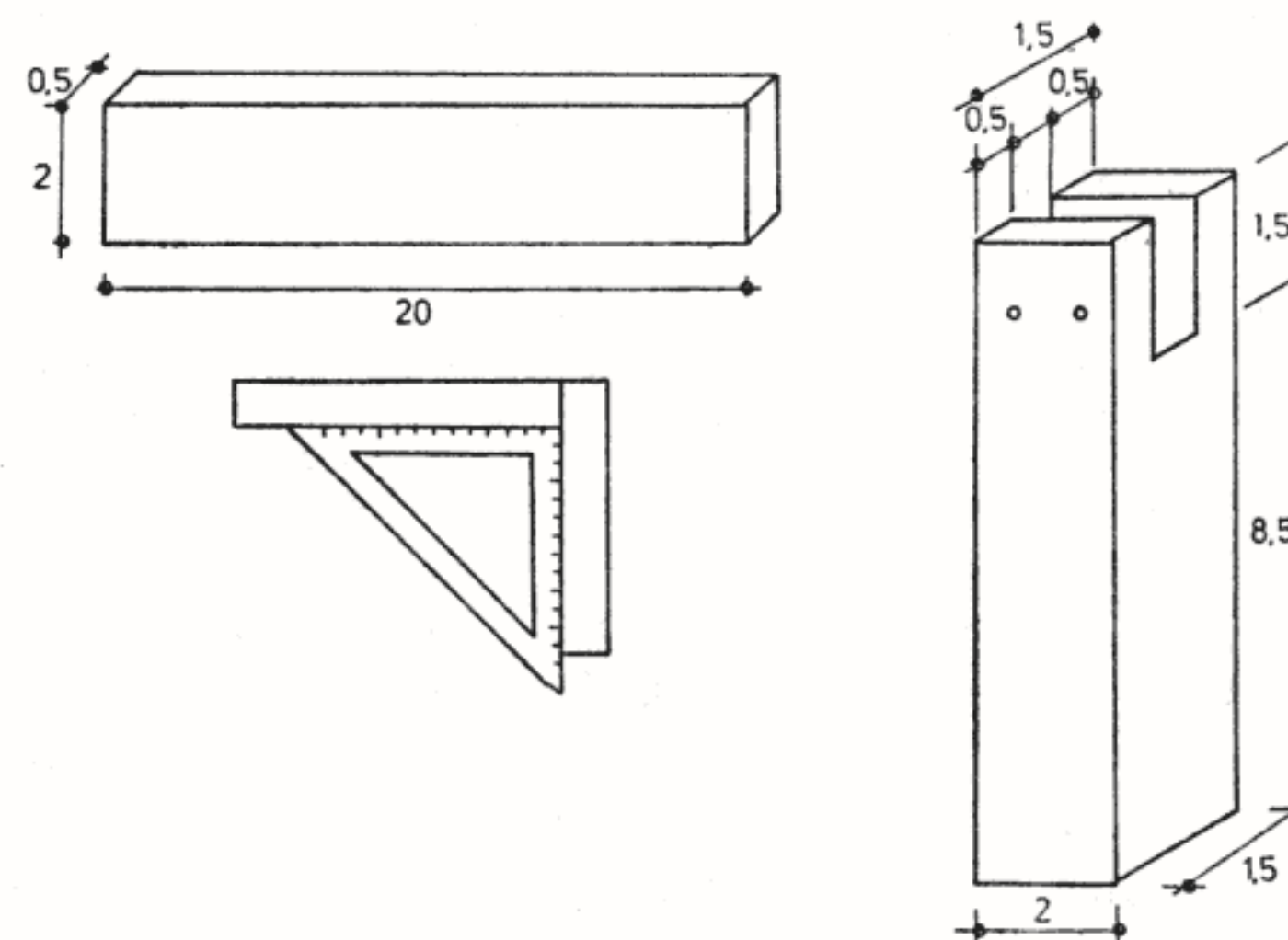
Fig. 20 — Echerul cu talpă
