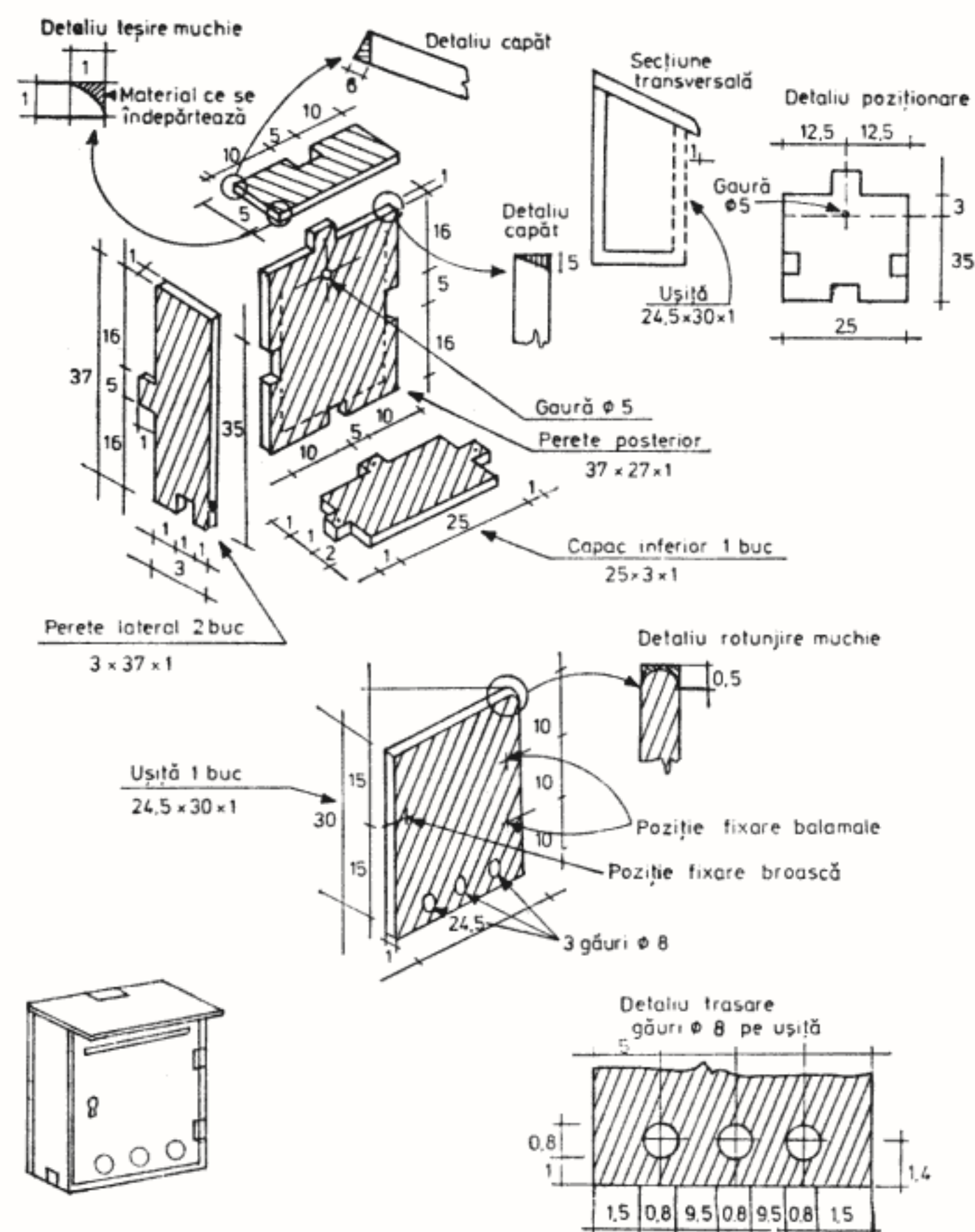
Fig. 39 — Cutie de scrisori
