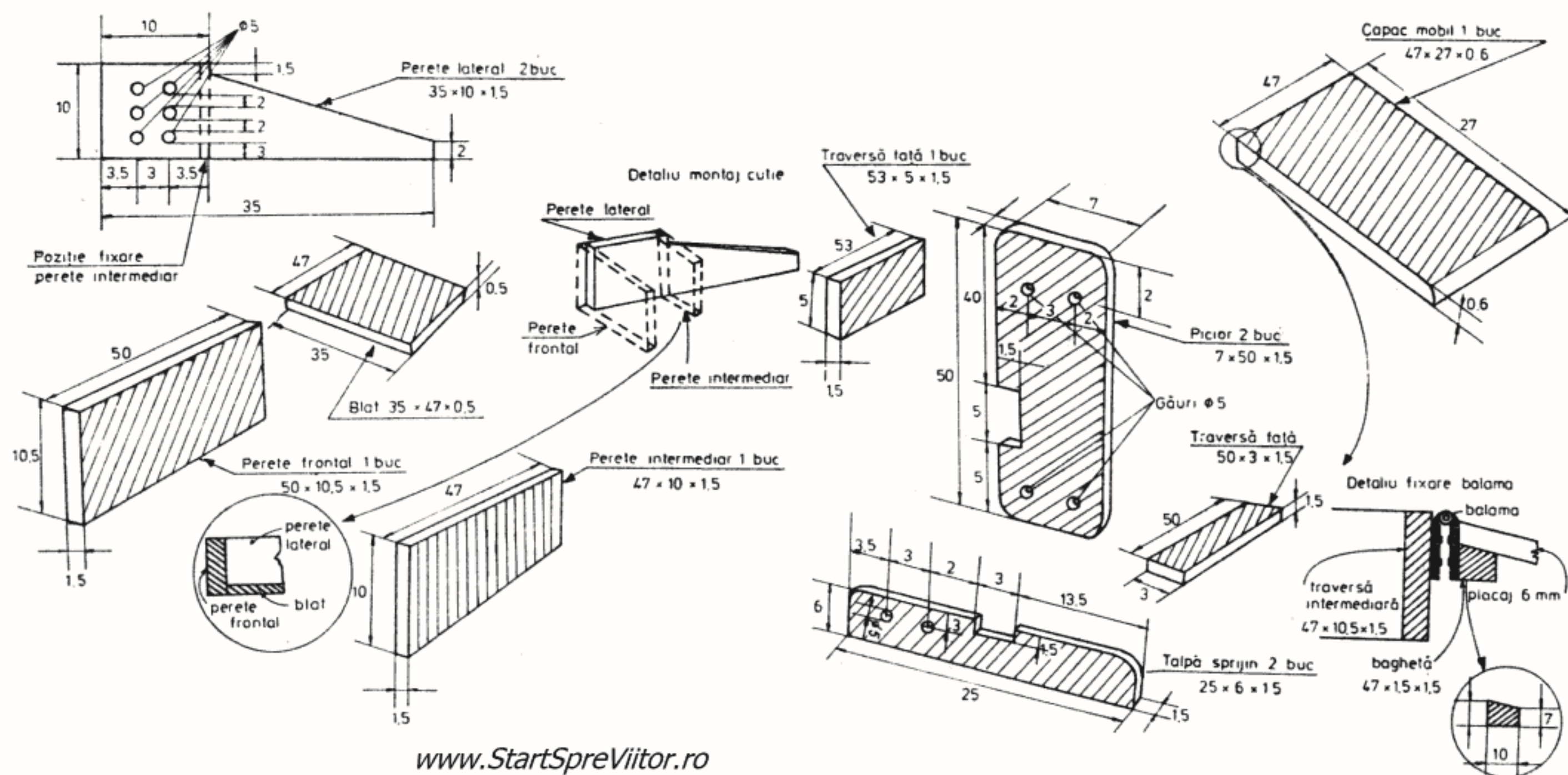
Fig. 34 — Măsuță reglabilă
