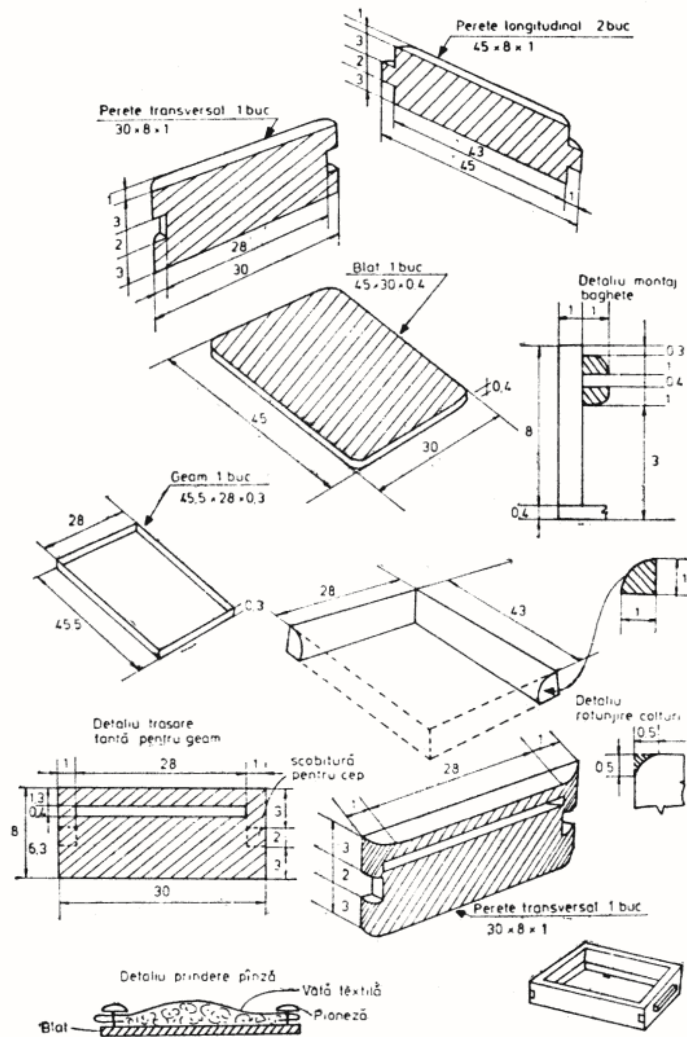
Fig. 31 — Cutie pentru insectar
