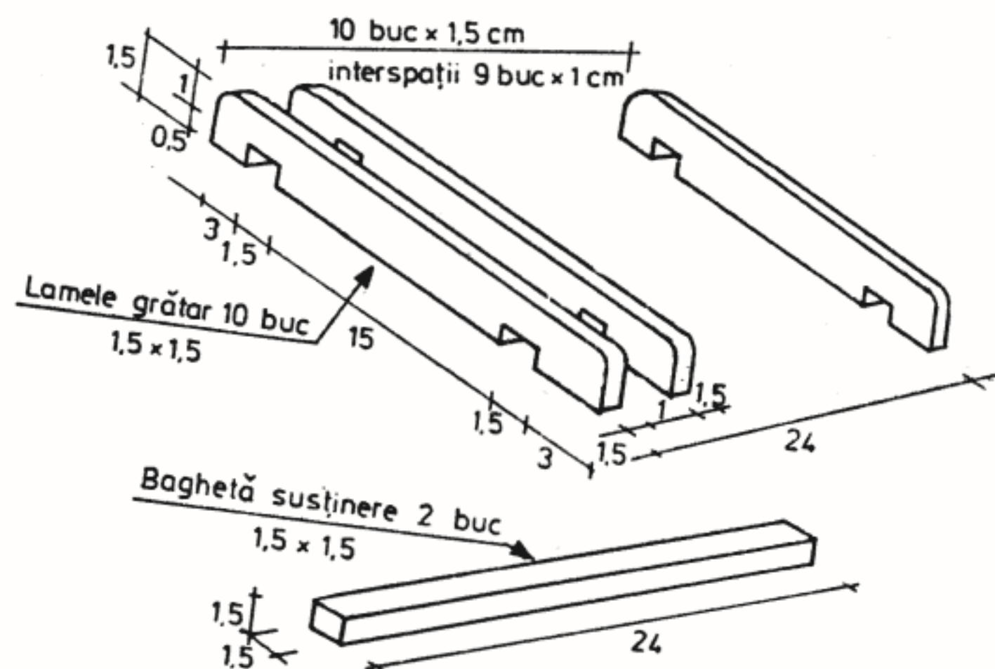
Fig. 36 — Grătar de lemn pentru spălător
