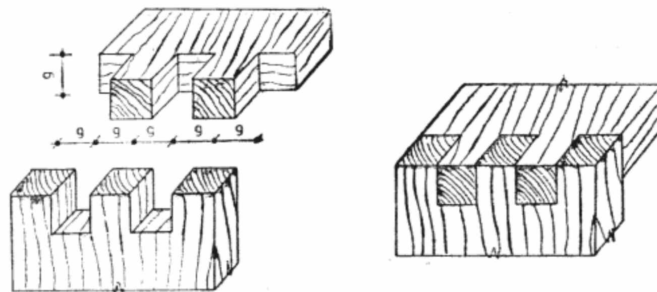
Fig. 8 — Îmbinare de colț cu cep multiplu
