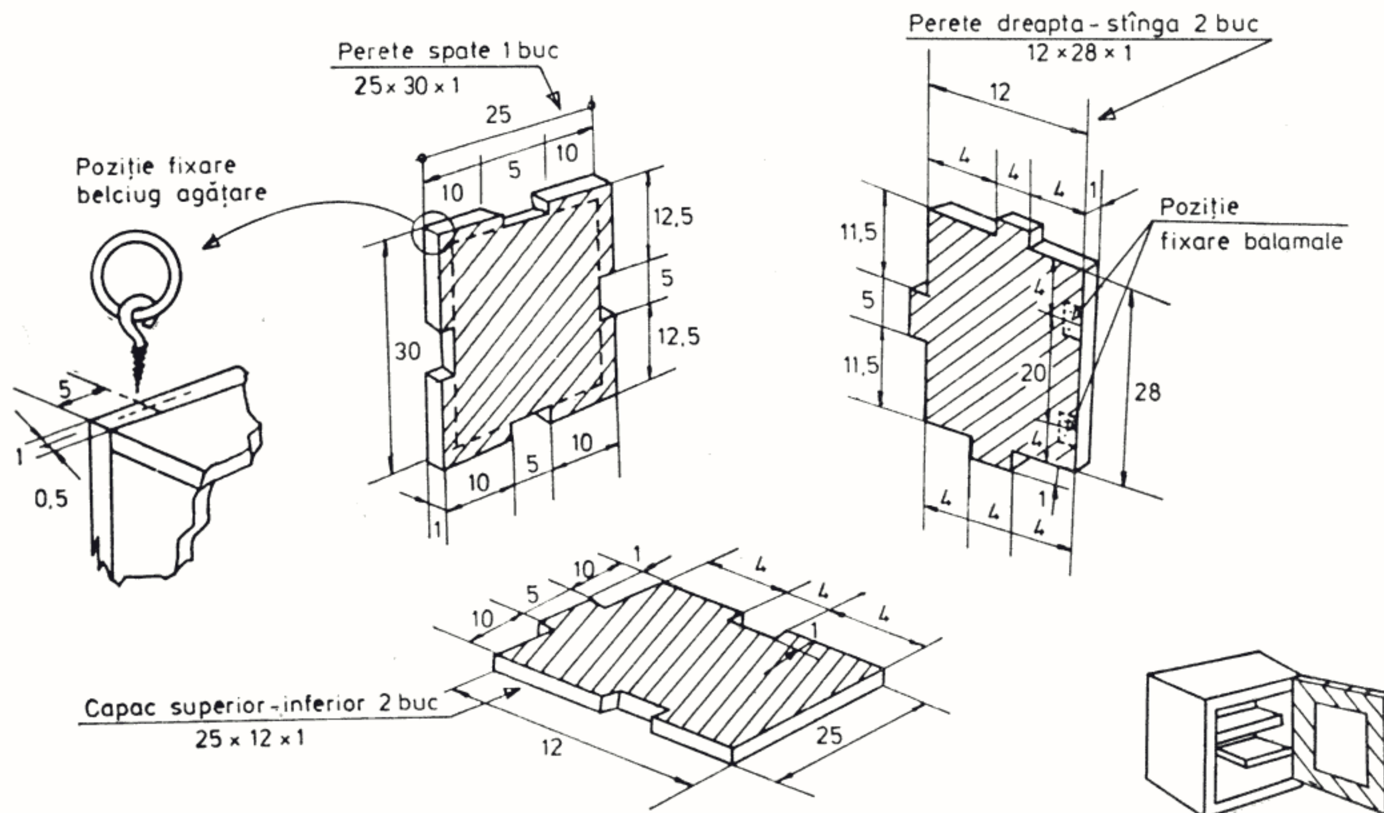
Fig. 41 b — Dulăpior pentru medicamente (detaliu pereți)
