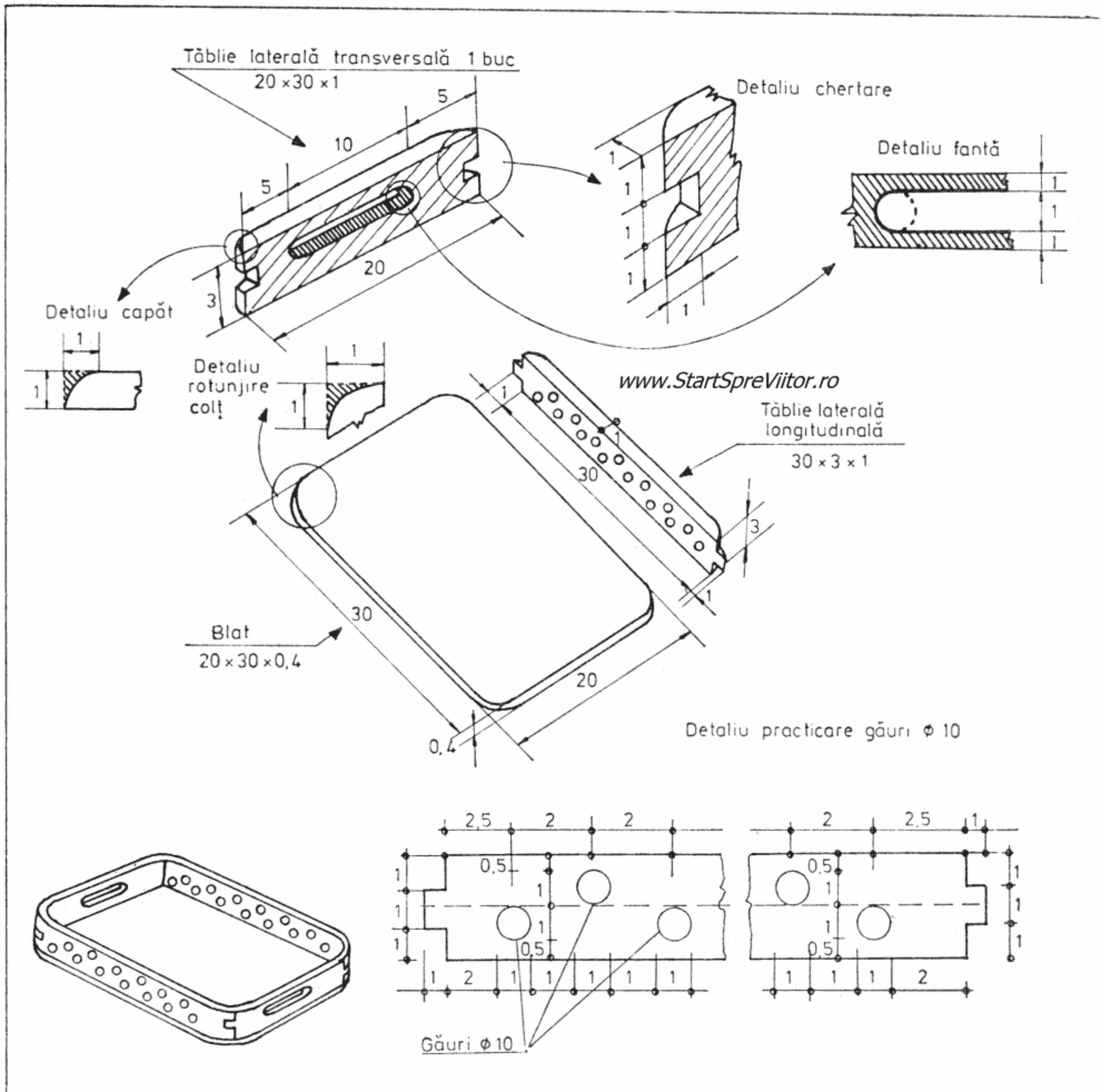
Fig. 40 — Tavă pentru fructe
