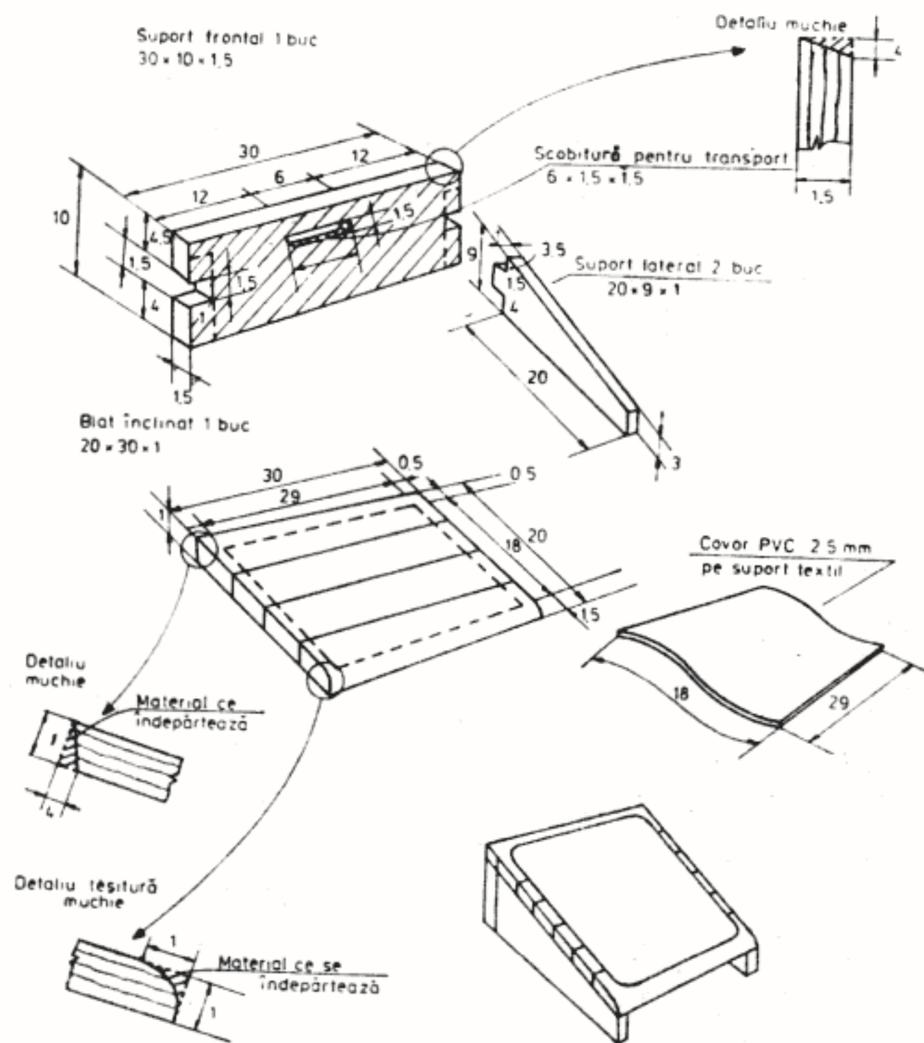
Fig. 25 — Suport pentru picioare
