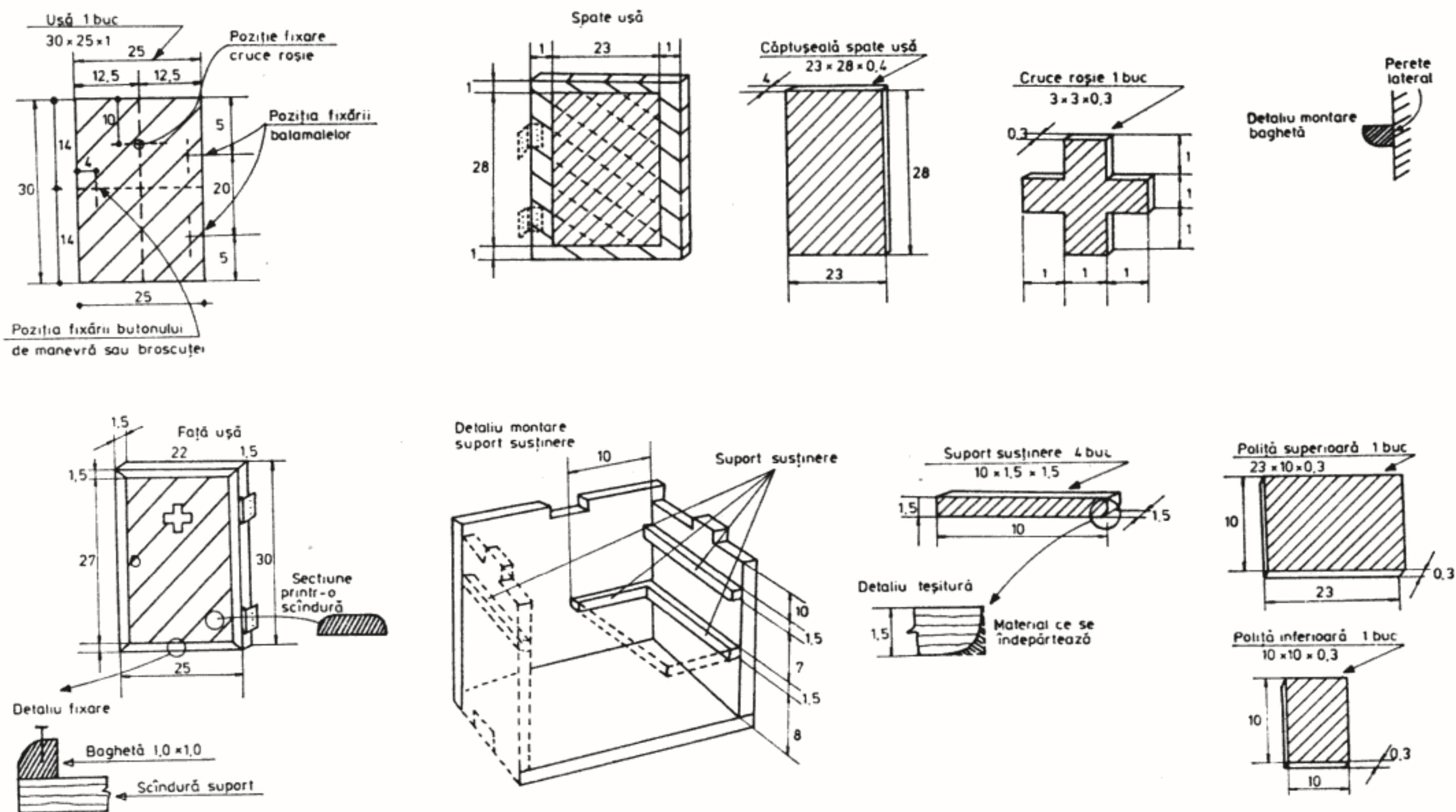
Fig. 41 a — Dulăpior pentru medicamente (detaliu ușă și suport susținere)
