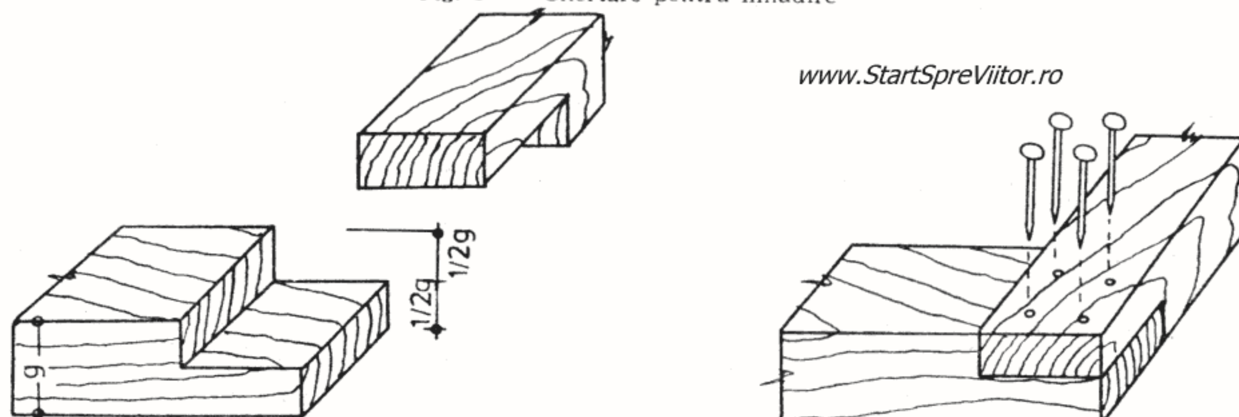
Fig. 2 — Chertare în unghi drept
