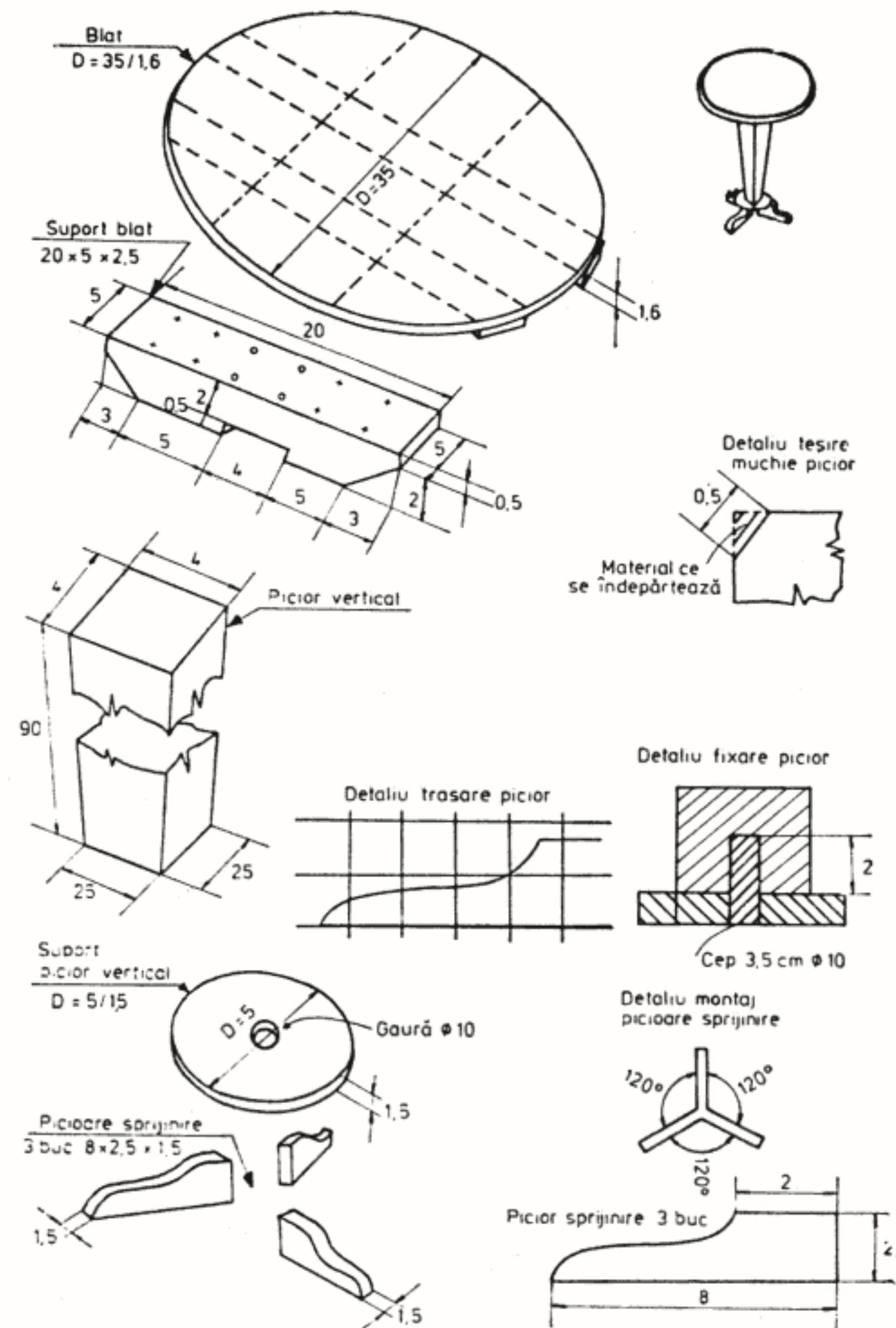
Fig. 32 — Măsuță pentru telefon
