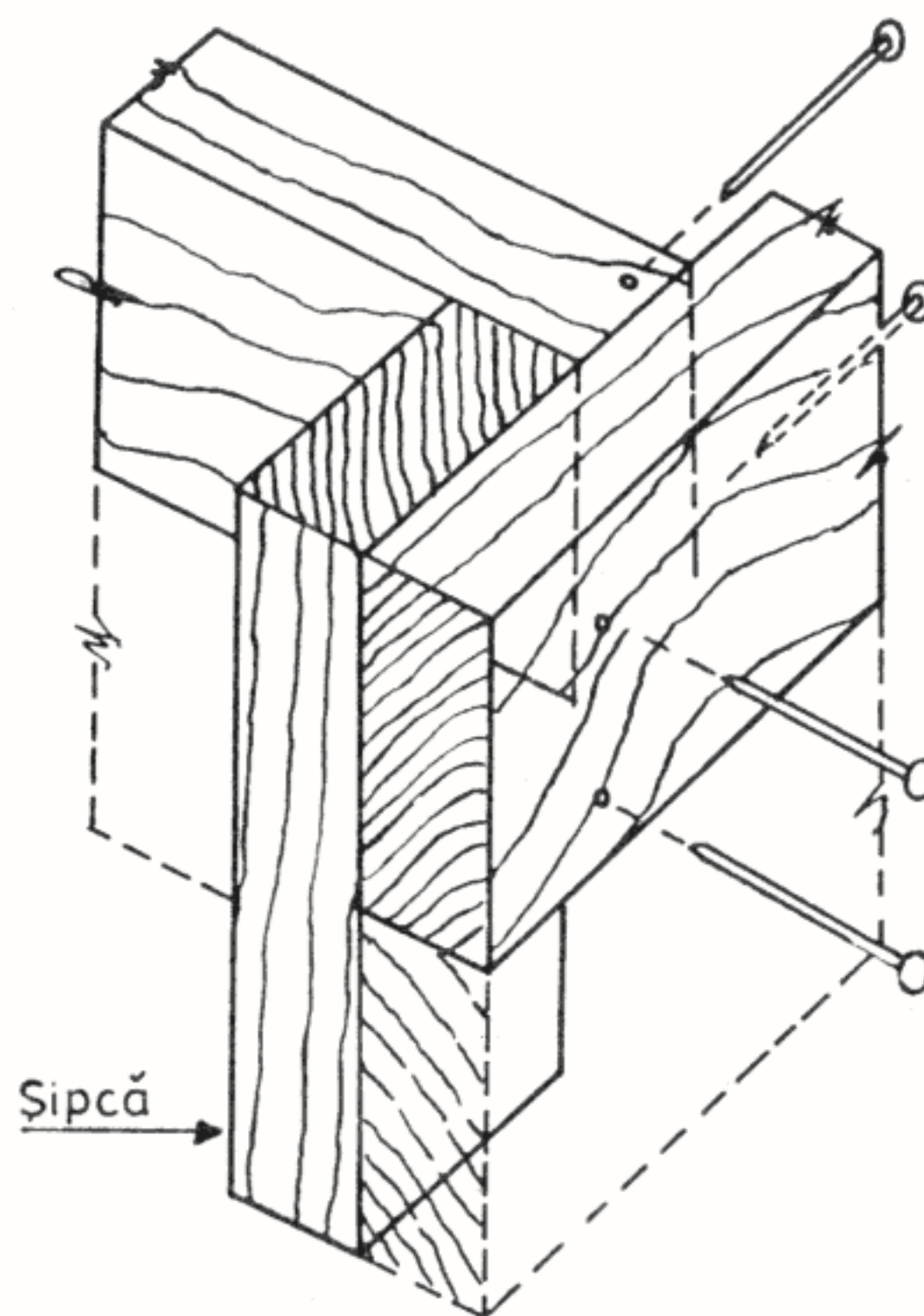
Fig. 11 — Îmbinare de colț cu șipcă exterioară
