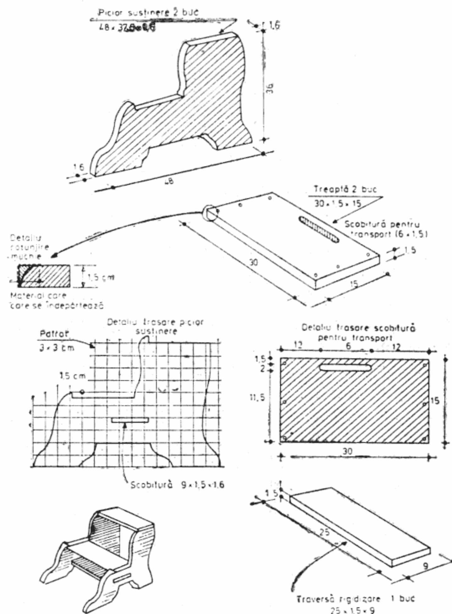
Fig. 26 — Scăriță pentru bibliotecă
