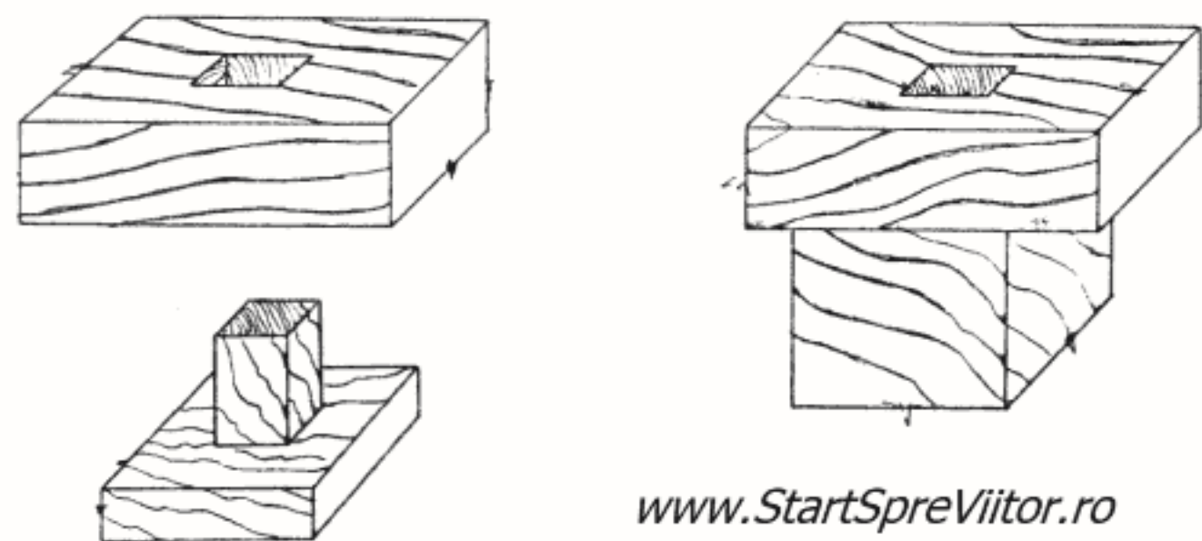
Fig. 7 — Îmbinare format T cu cep străpuns
