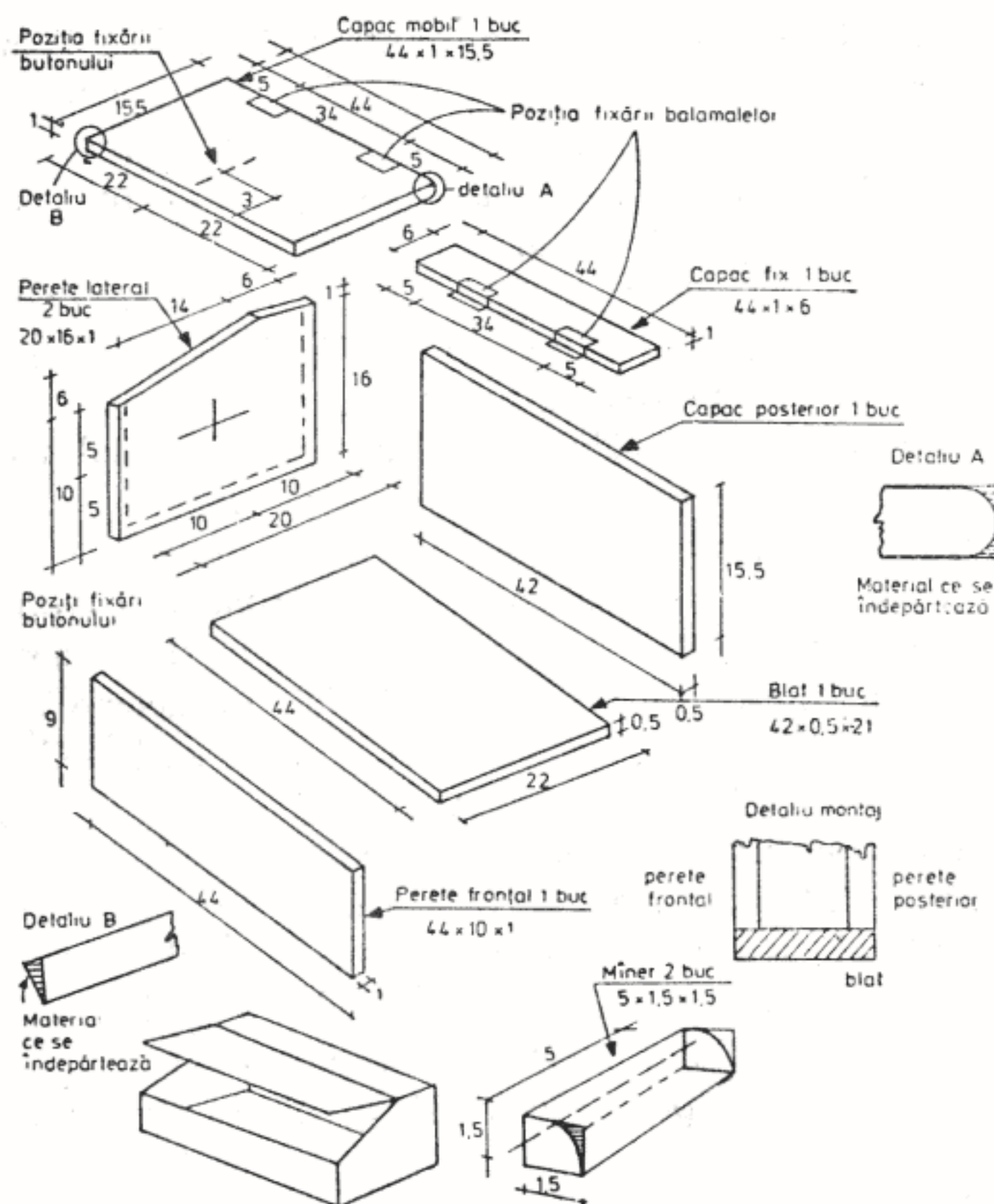
Fig. 24 — Cutie pentru păstrat plinea
