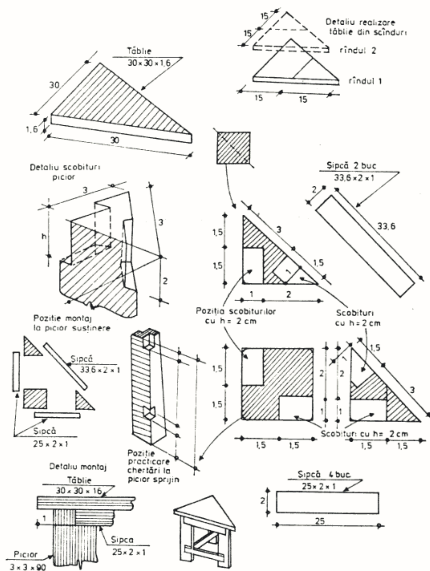
Fig. 33 — Măsuță de colț
