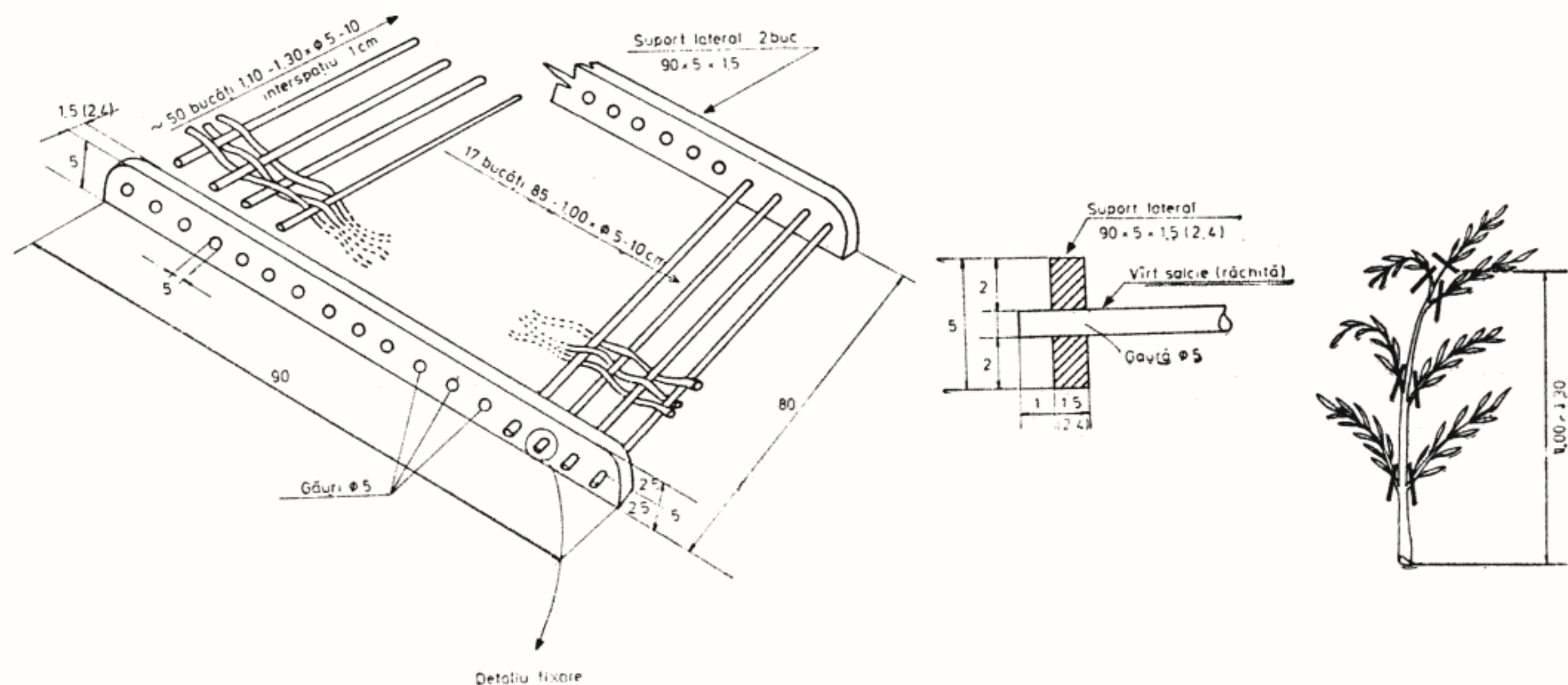
Fig. 38 — Uscător de fructe
